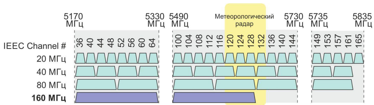
Рисунок 26. Wi-Fi-каналы 5 ГГц
