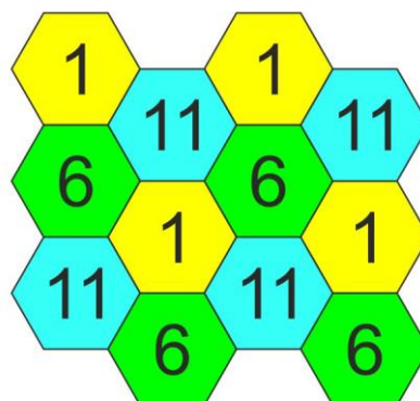
Рисунок 25. Схема распределения каналов между соседними точками доступа
