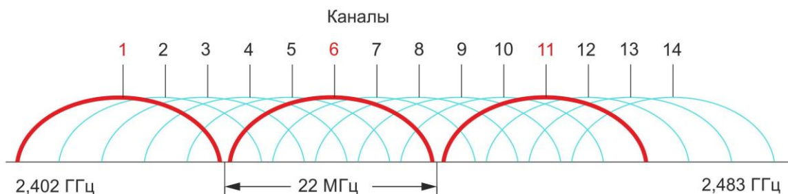
Рисунок 24. Wi-Fi-каналы 2,4 ГГц
