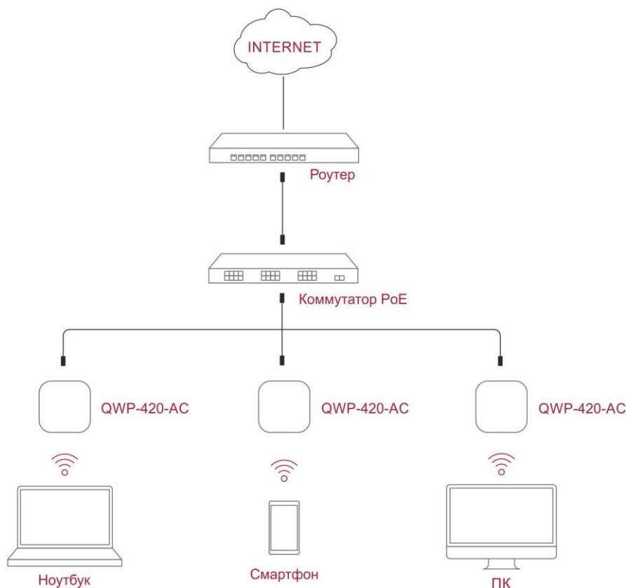
Рисунок 1. Типовая схема подключения точек доступа к сетевому оборудованию
