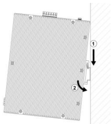
DIN-Rail монтаж
