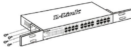
Рисунок 2. Крепление кронштейнов
