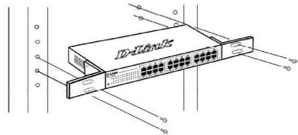
Рисунок 3. Установка коммутатора в стойку
