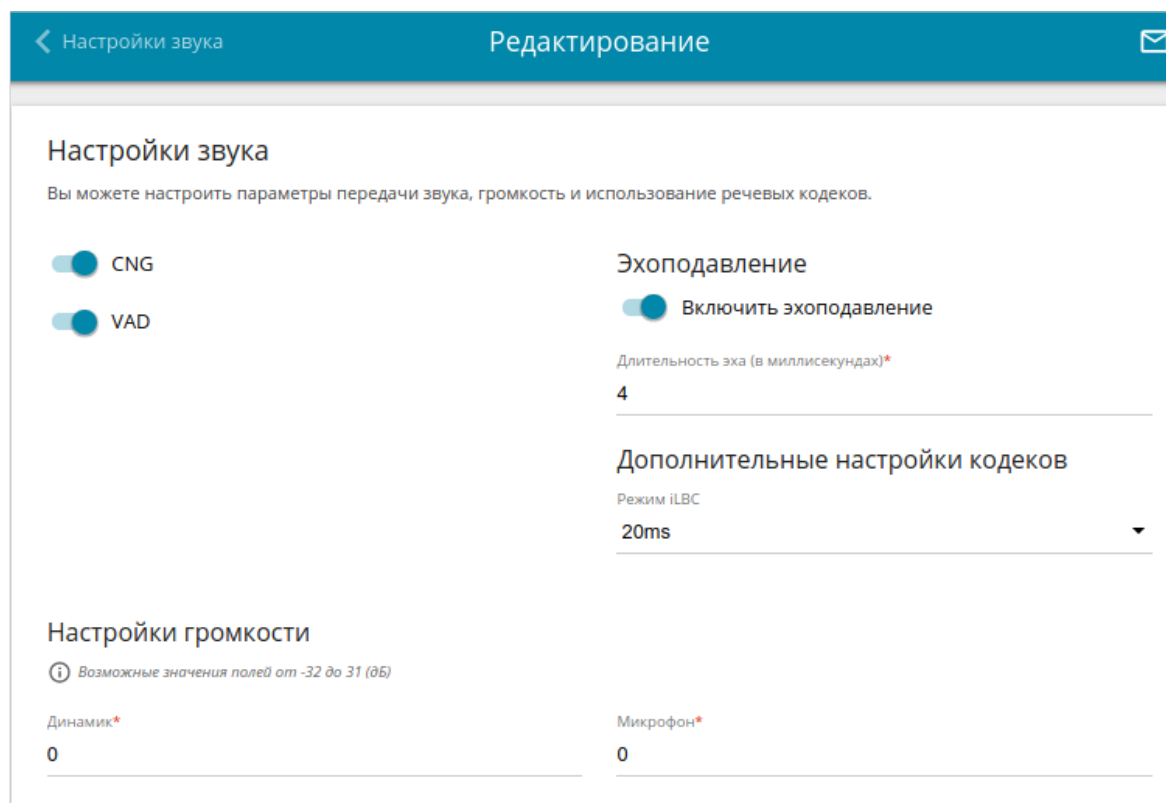
Рисунок 215. Страница редактирования настроек звука для линии.
