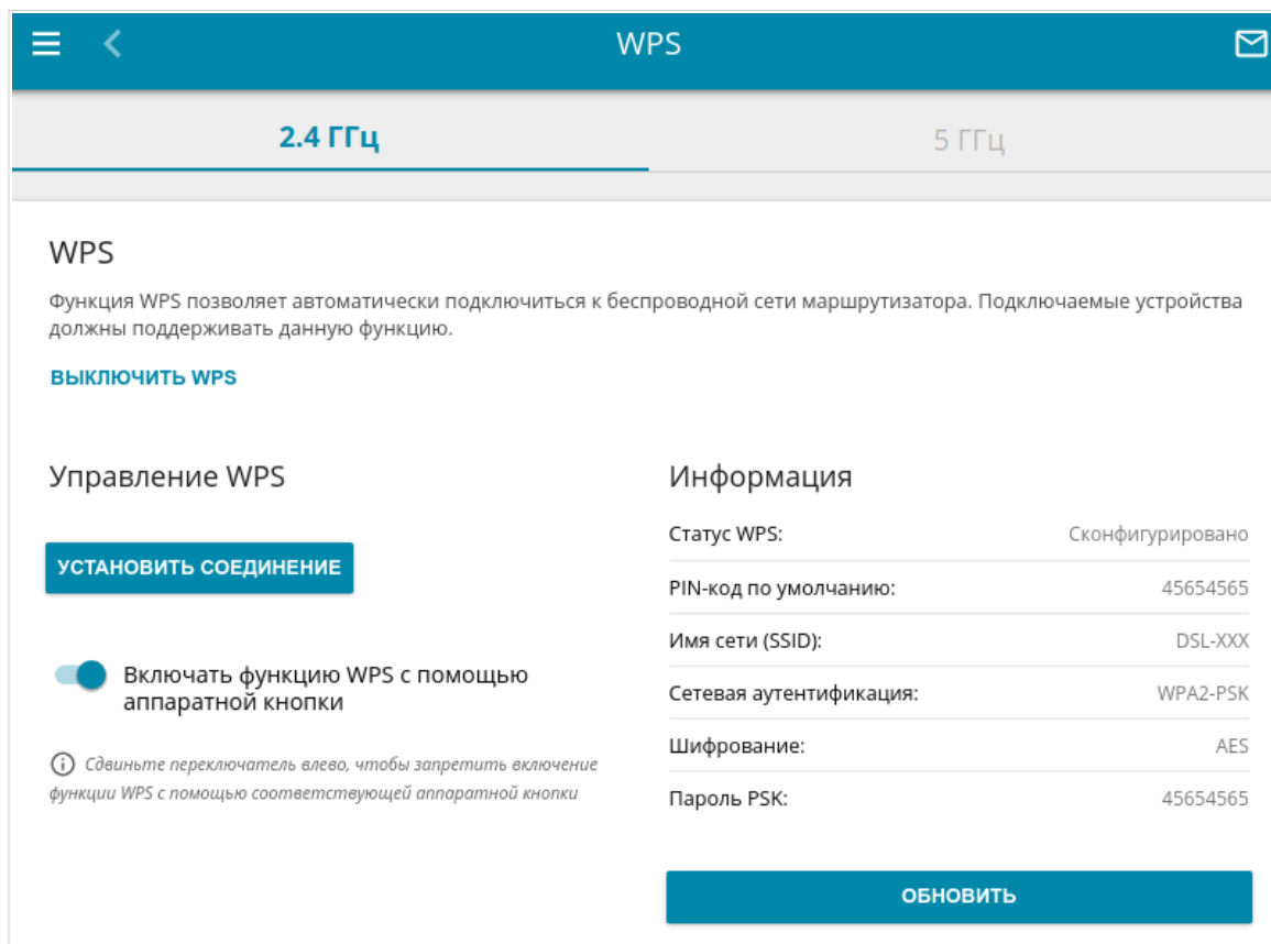
Рисунок 145. Страница для настройки функции WPS.
