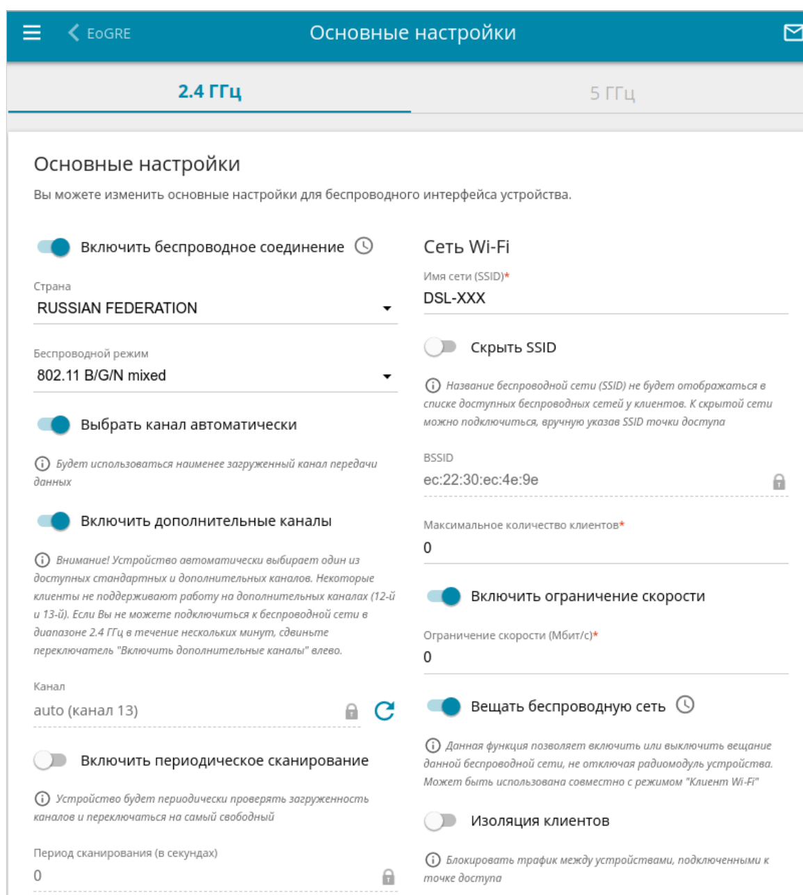
Рисунок 138. Основные настройки беспроводной локальной сети в диапазоне 2,4 ГГц.
