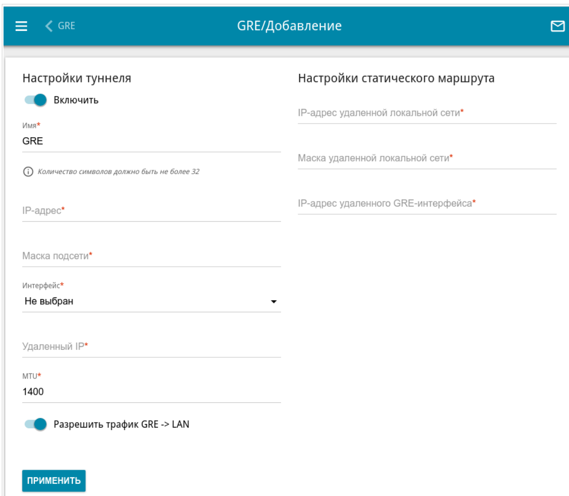
Рисунок 131. Страница добавления GRE-туннеля.
