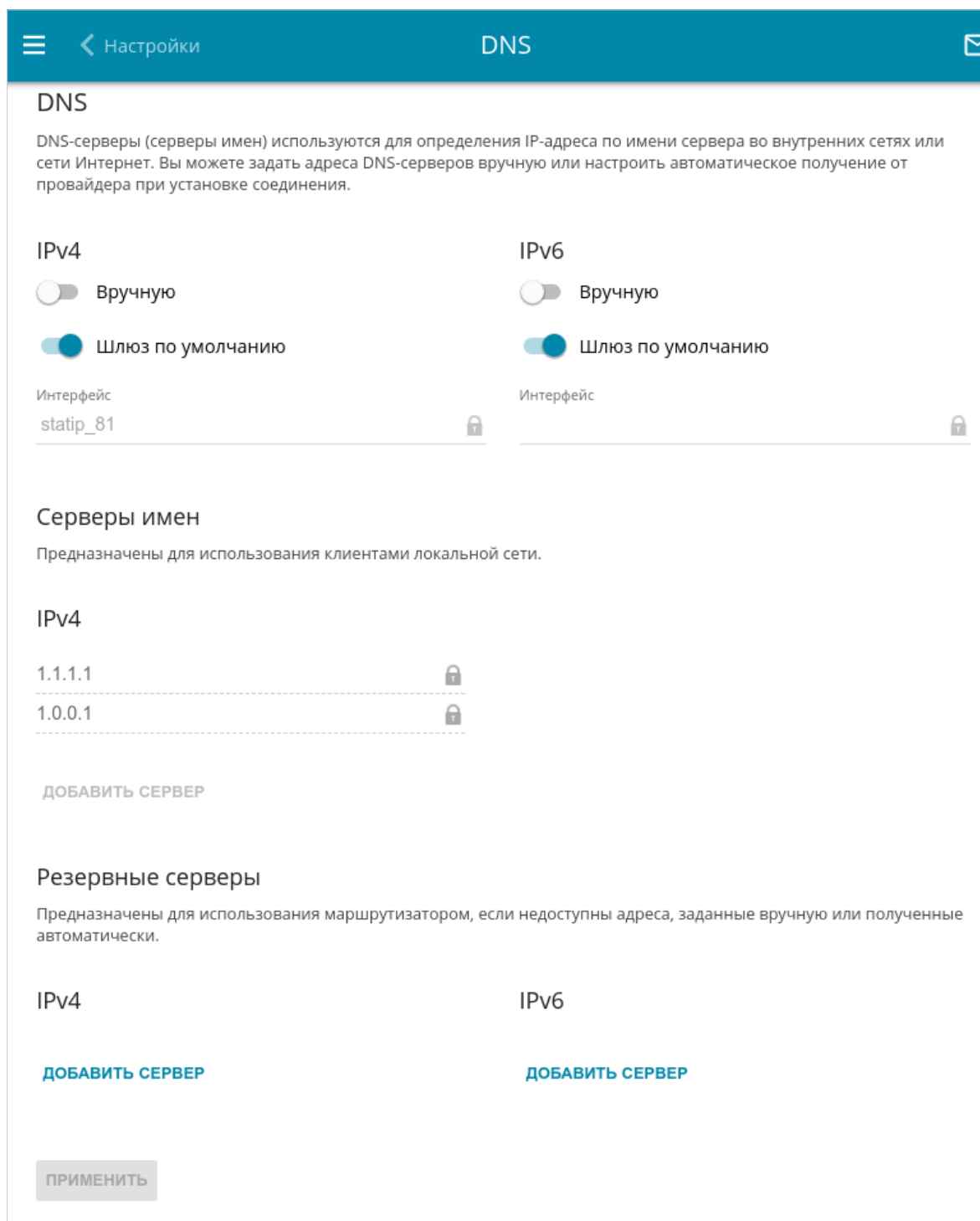
Рисунок 182. Страница Дополнительно / DNS .
