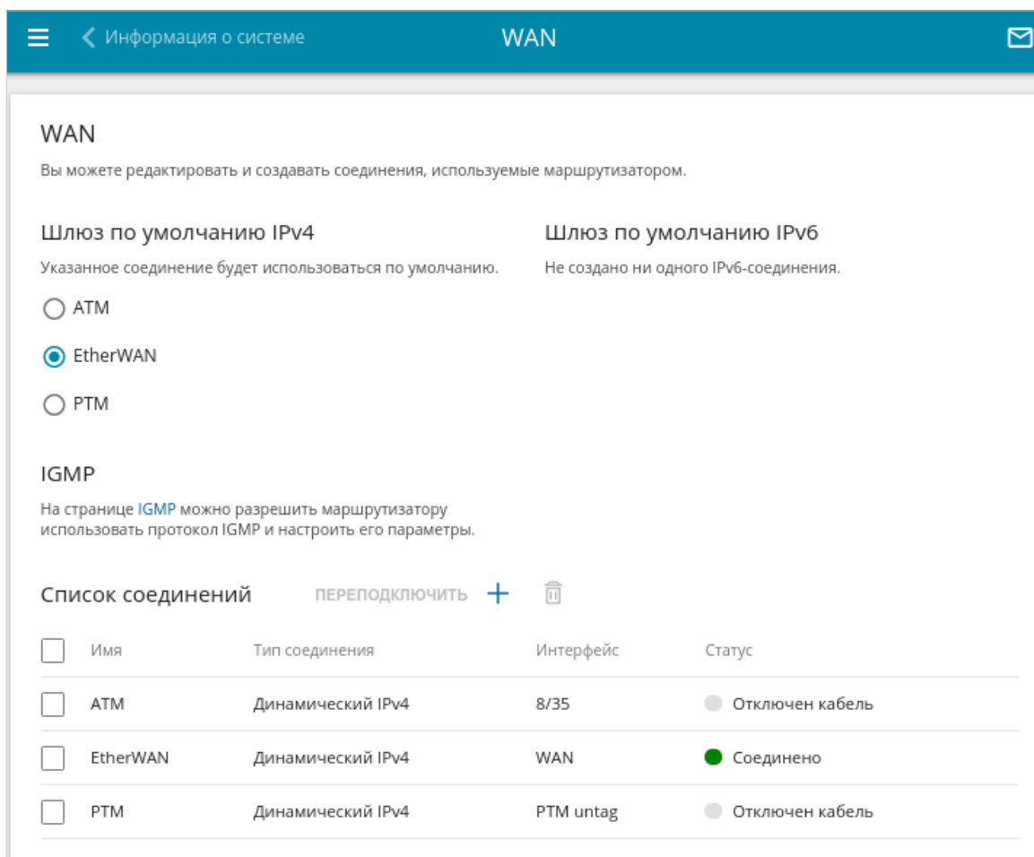
Рисунок 68. Страница Настройка соединений / WAN . Расширенный режим.
