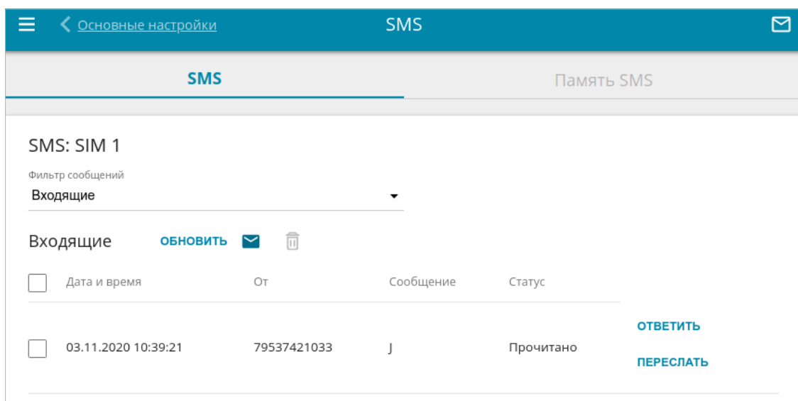
Рисунок 171. Страница USB-модем / Название модема / SMS . Вкладка SMS .
