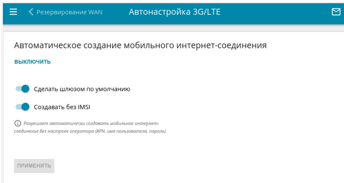
Рисунок 123. Страница Настройка соединений / Автонастройка 3G/LTE .
