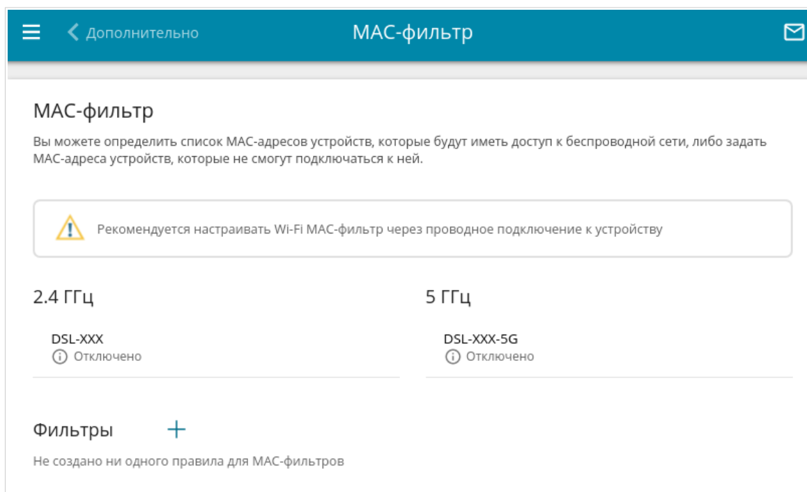
Рисунок 152. Страница для настройки MAC-фильтра для беспроводной сети.
