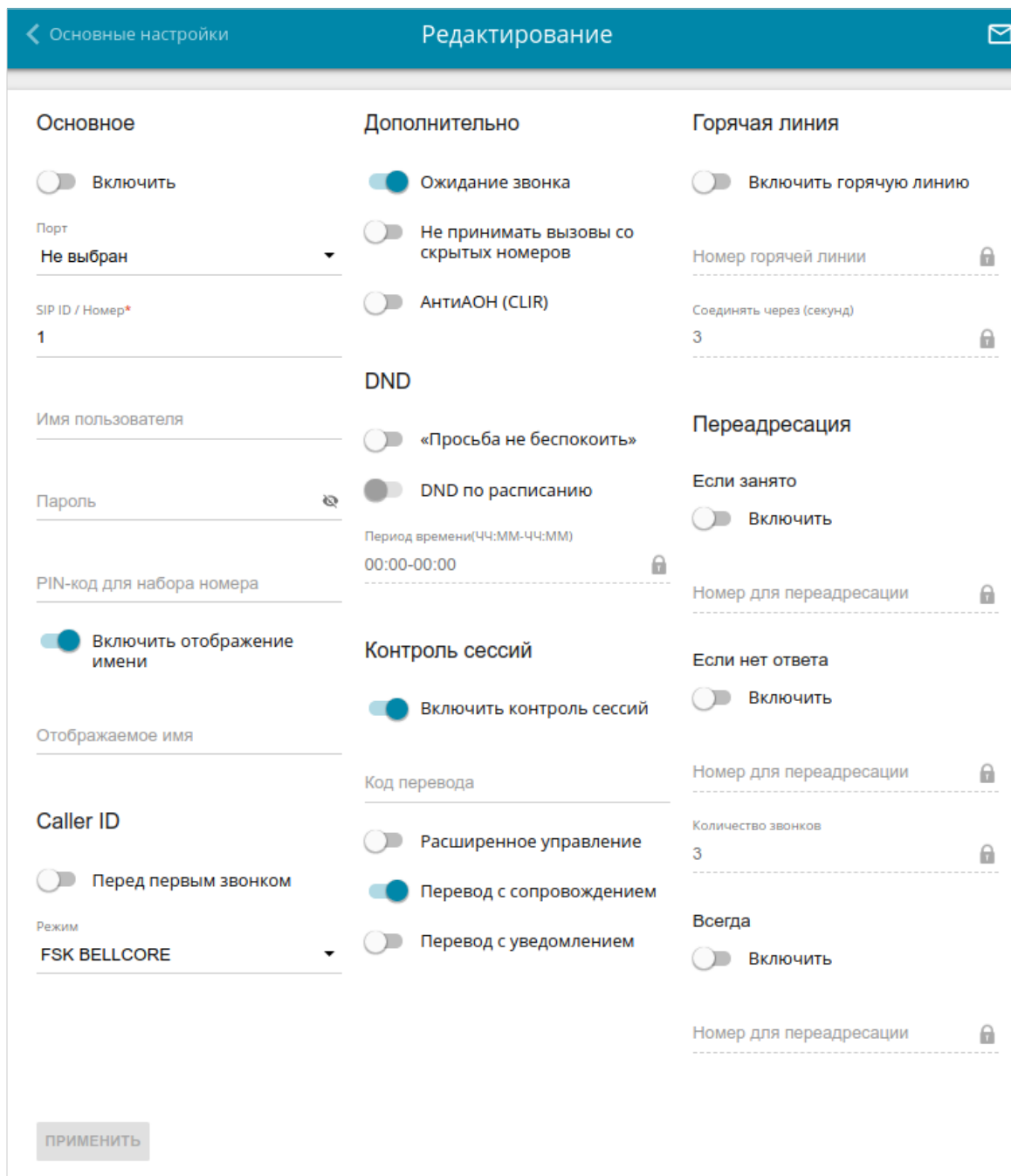
Рисунок 208. Страница изменения параметров SIP-линии.
