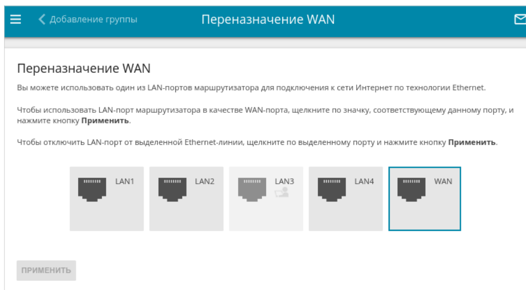
Рисунок 179. Страница Дополнительно / Переназначение WAN .
