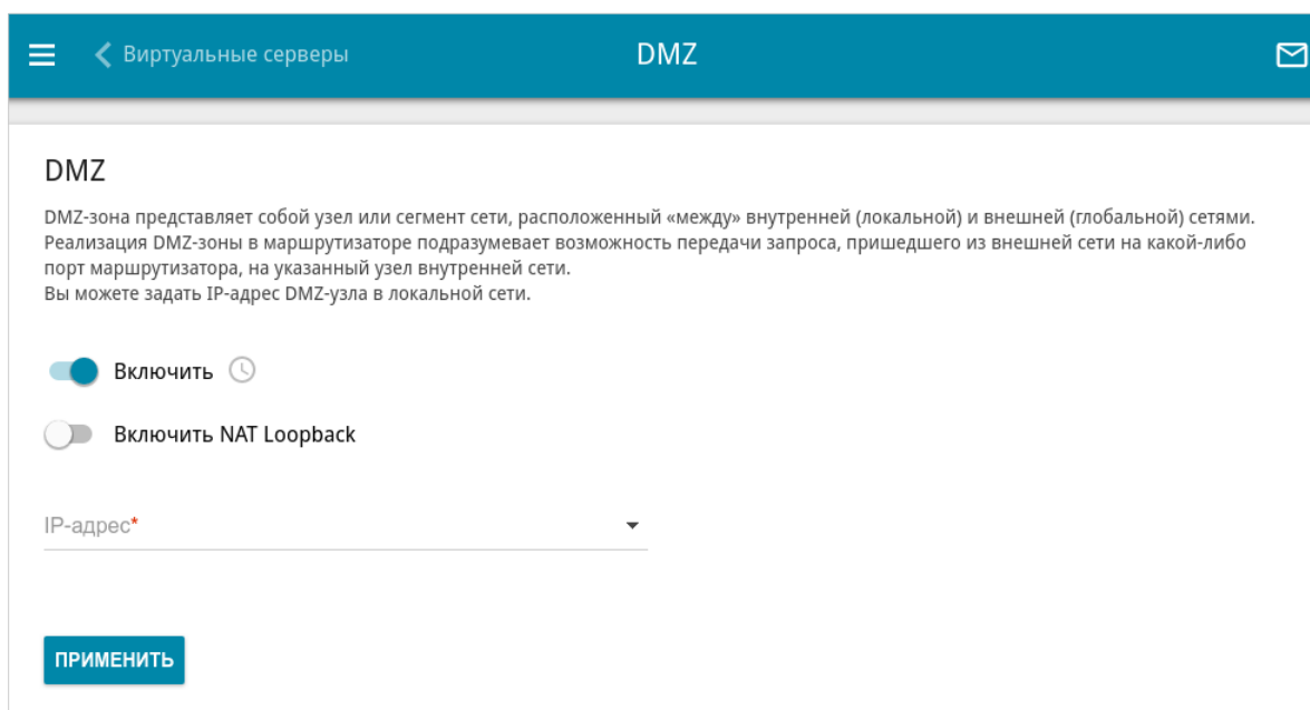
Рисунок 227. Страница Межсетевой экран / DMZ .
