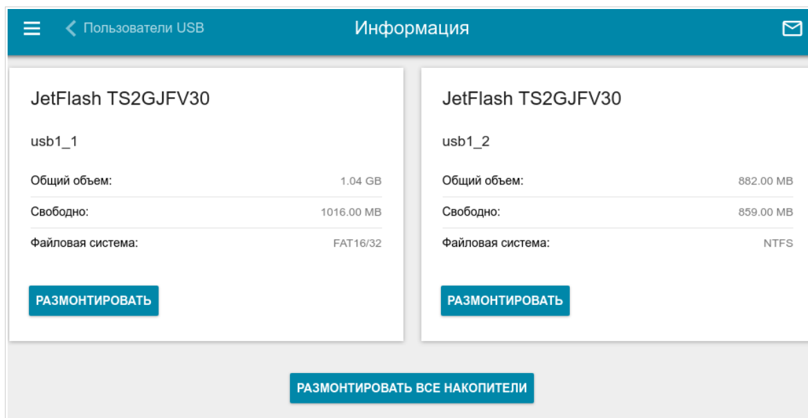
Рисунок 156. Страница USB-накопитель / Информация .
