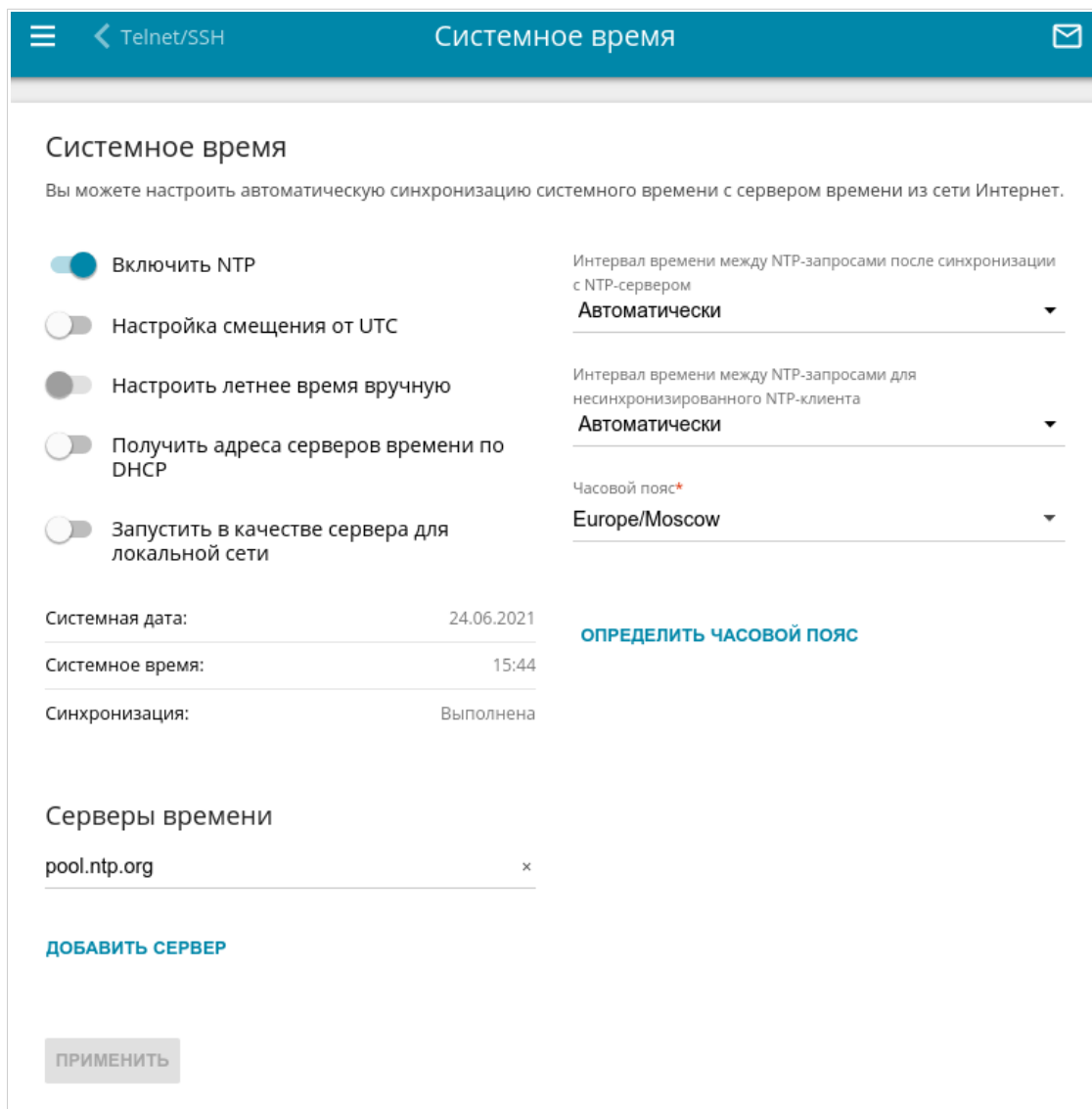
Рисунок 245. Страница Система / Системное время .
