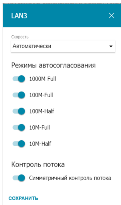
Рисунок 186. Окно изменения настроек порта маршрутизатора.
