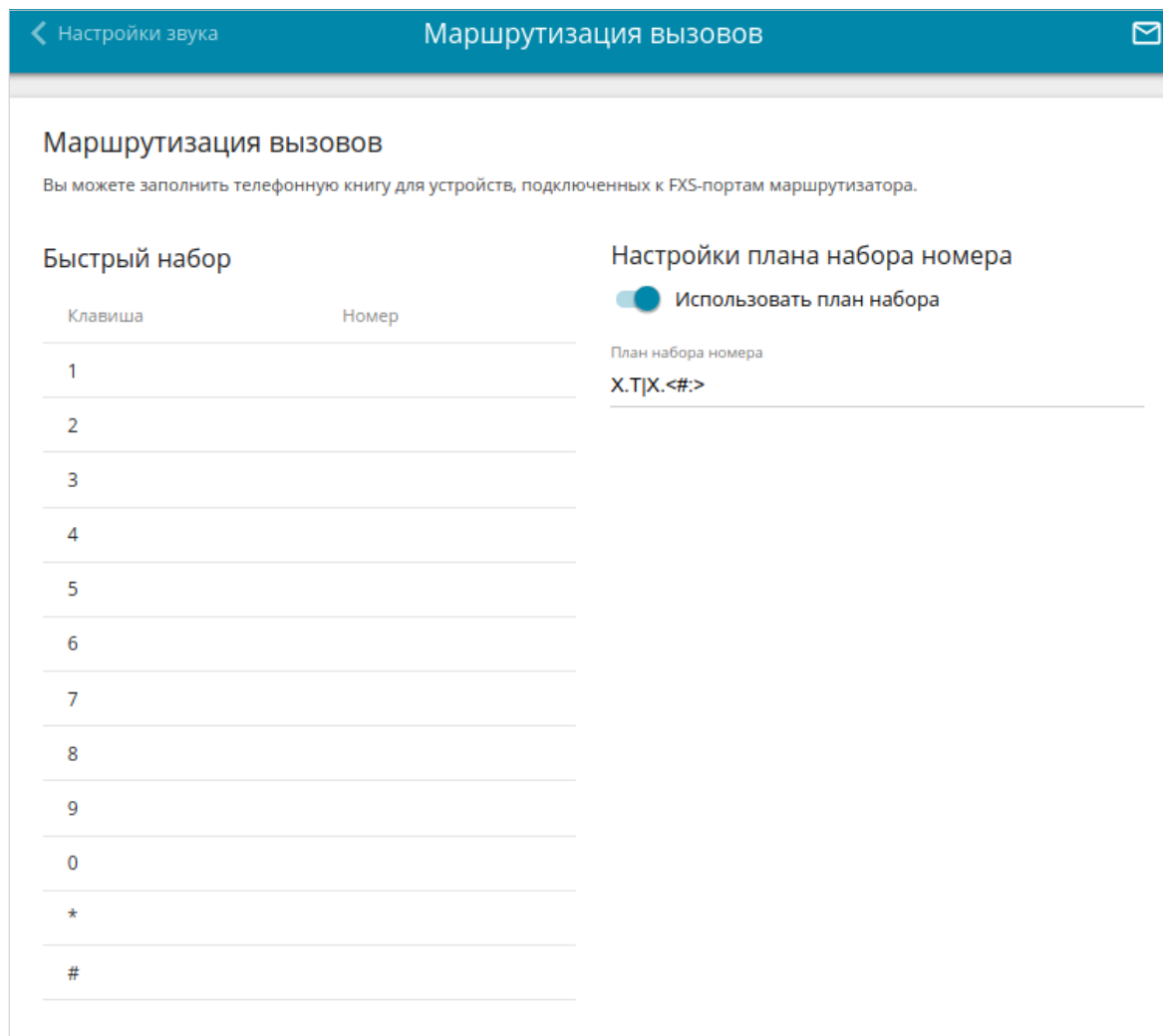
Рисунок 218. Страница VoIP / Имя профиля / Маршрутизация вызовов .
