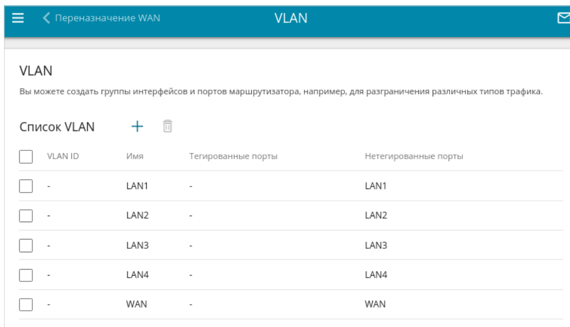
Рисунок 175. Страница Дополнительно / VLAN .
