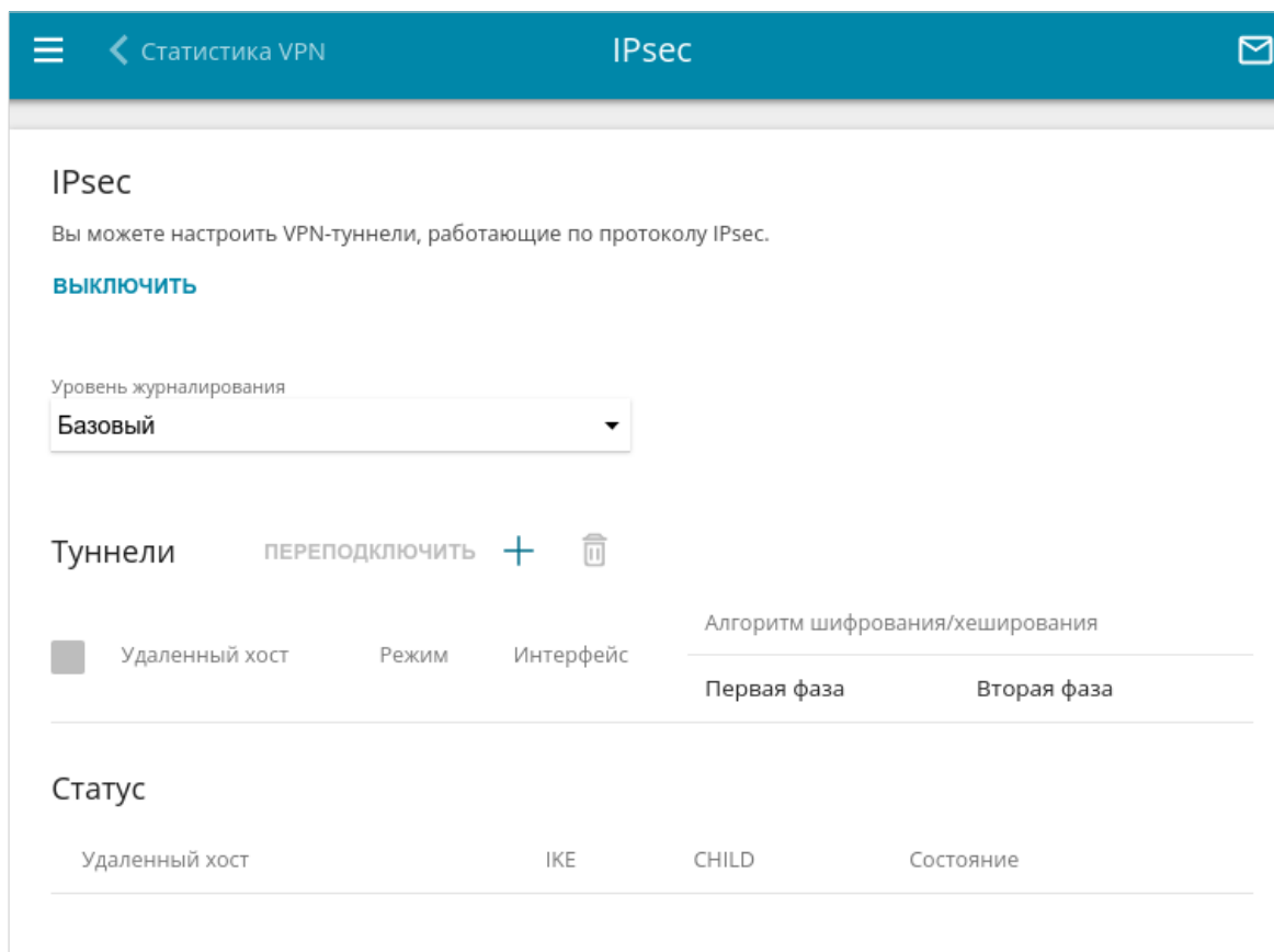
Рисунок 126. Страница VPN / IPsec.
