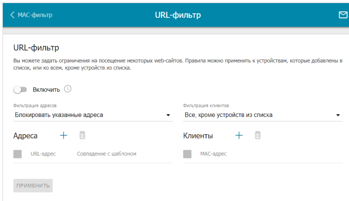
Рисунок 230. Страница Межсетевой экран / URL-фильтр .
