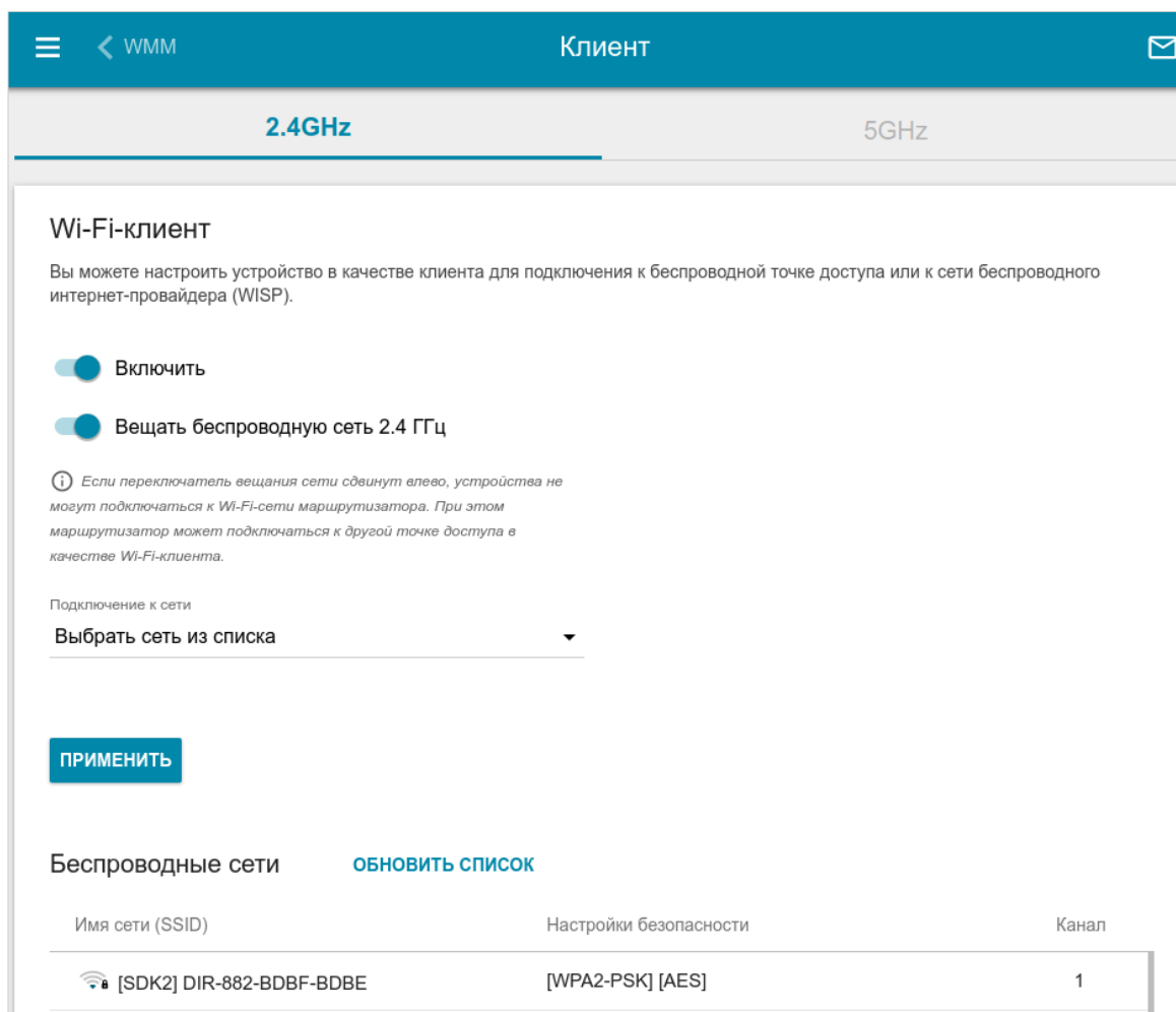
Рисунок 148. Страница для настройки маршрутизатора в качестве клиента.
