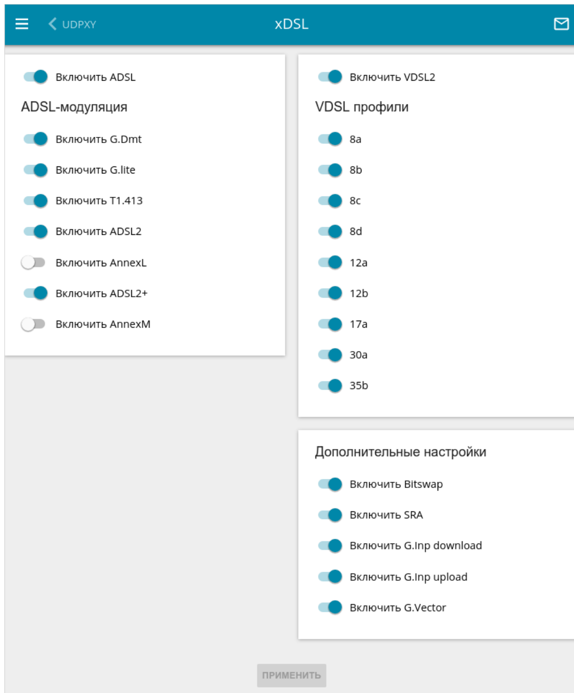
Рисунок 195. Страница Дополнительно / xDSL .
