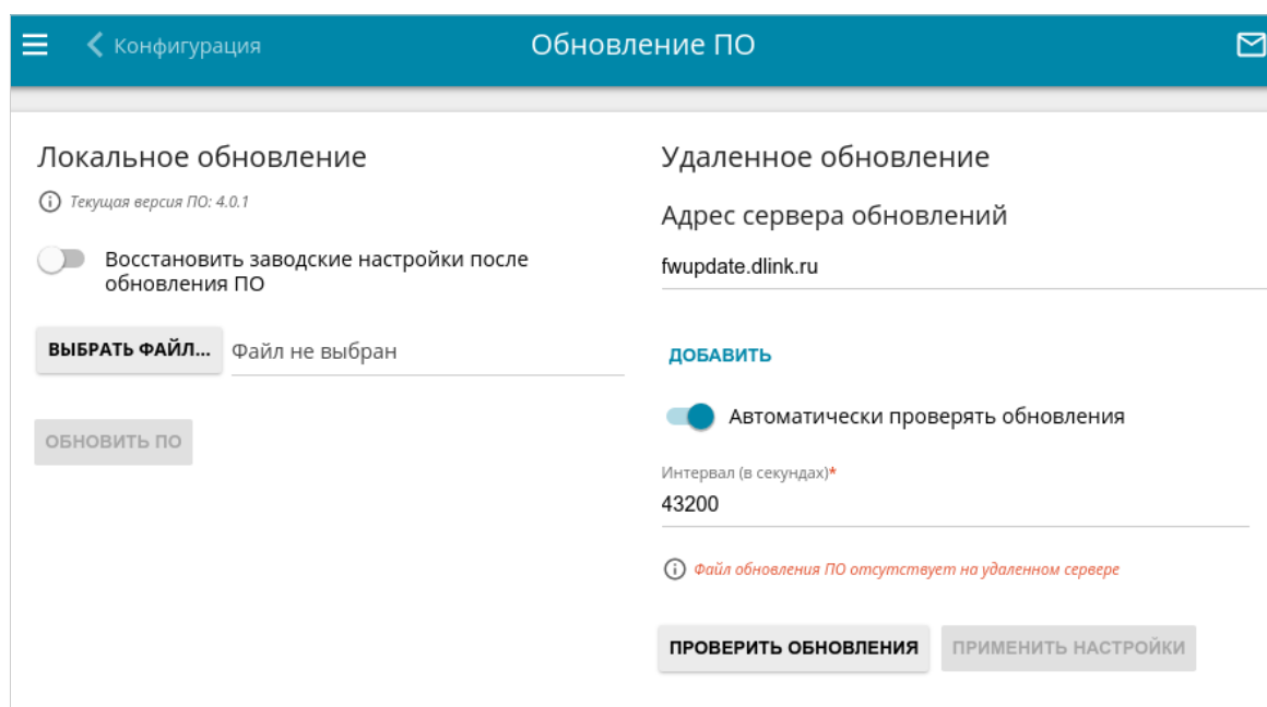
Рисунок 234. Страница Система / Обновление ПО .
