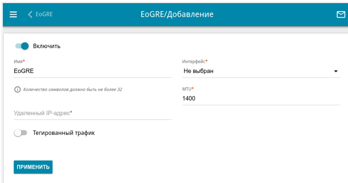
Рисунок 137. Страница добавления ЕоGRE-туннеля.
