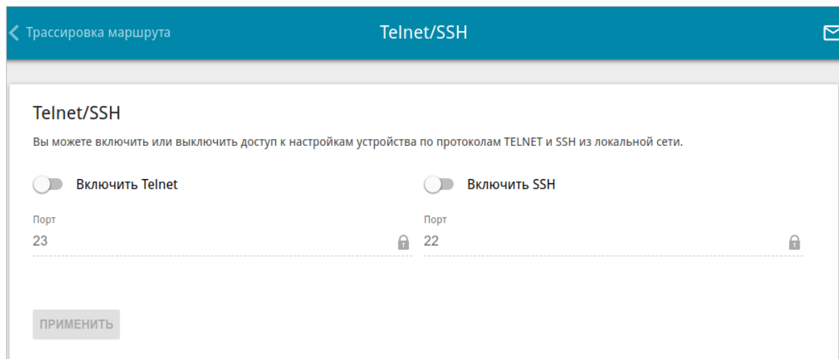
Рисунок 244. Страница Система / Telnet/SSH .
