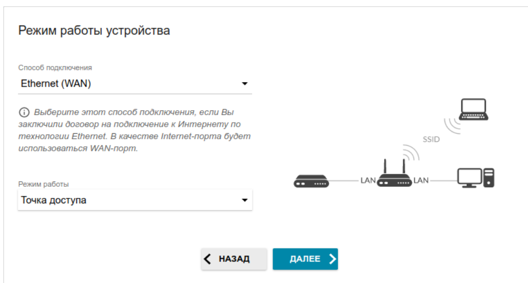
Рисунок 38. Выбор режима работы устройства. Режим Точка доступа.
