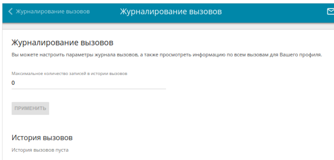
Рисунок 222. Страница VoIP / Имя профиля / Журналирование вызовов . Данные линии.
