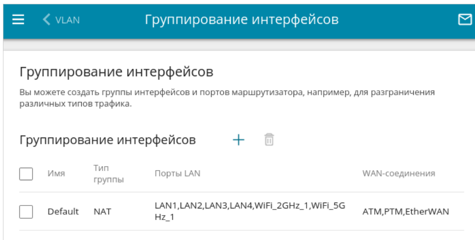
Рисунок 177. Страница Дополнительно / Группирование интерфейсов .
