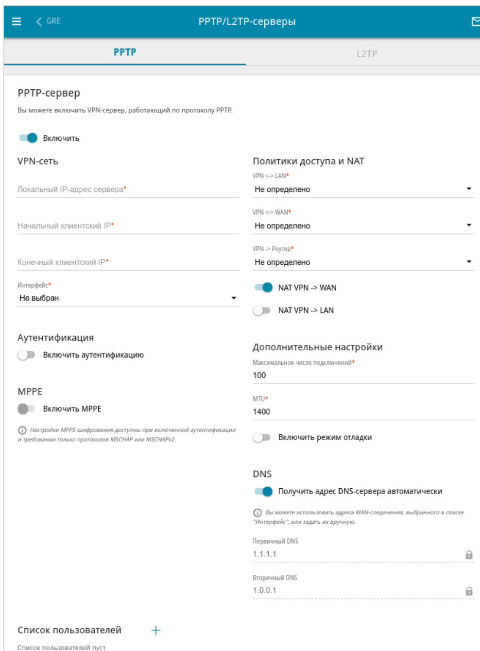
Рисунок 132. Страница VPN / PPTP/L2TP-серверы .
