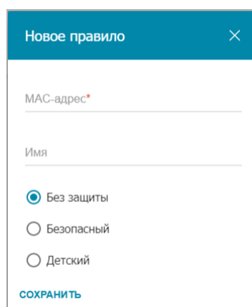
Рисунок 249. Добавление правила для сервиса Яндекс.DNS.
