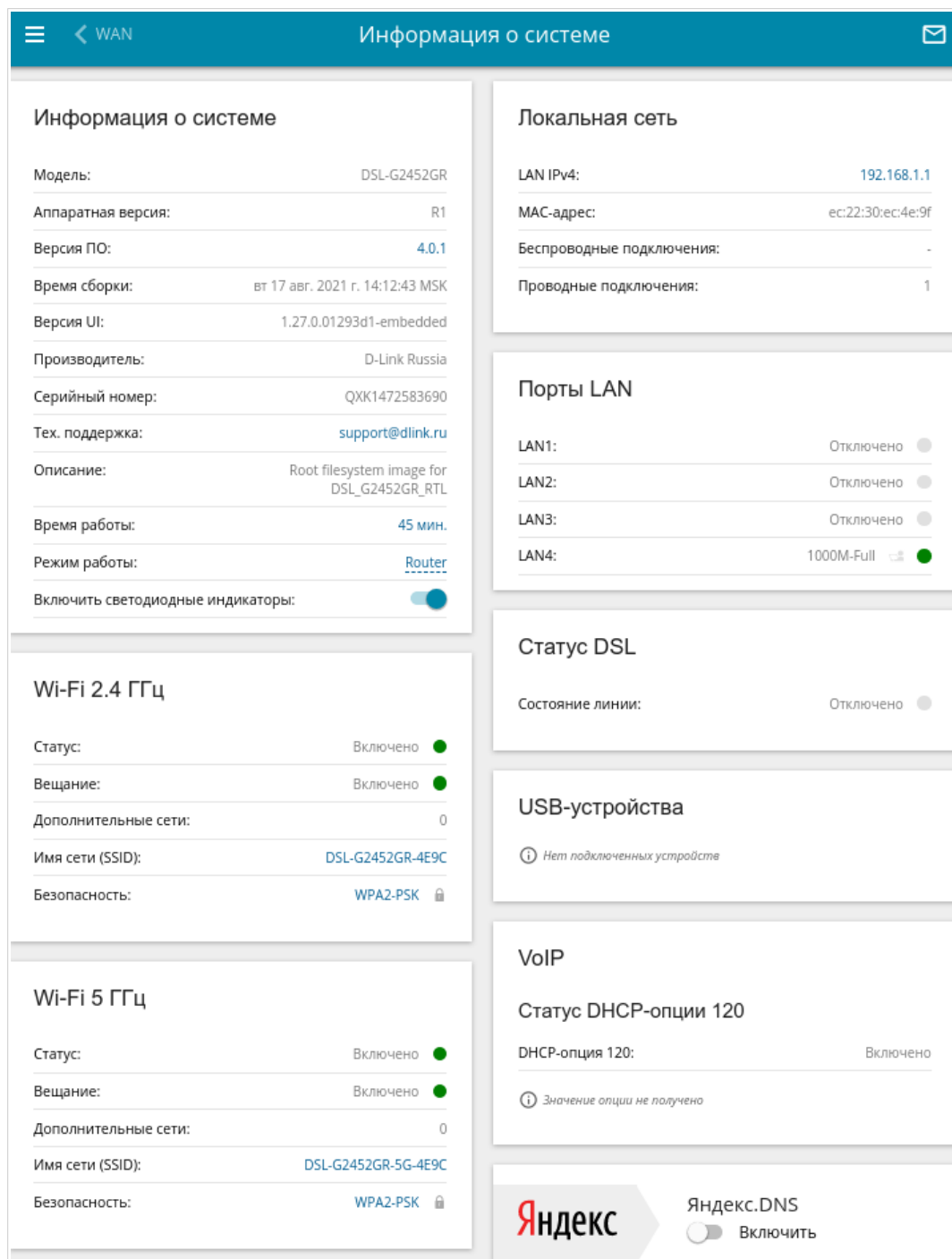
Рисунок 26. Страница информации о системе.
