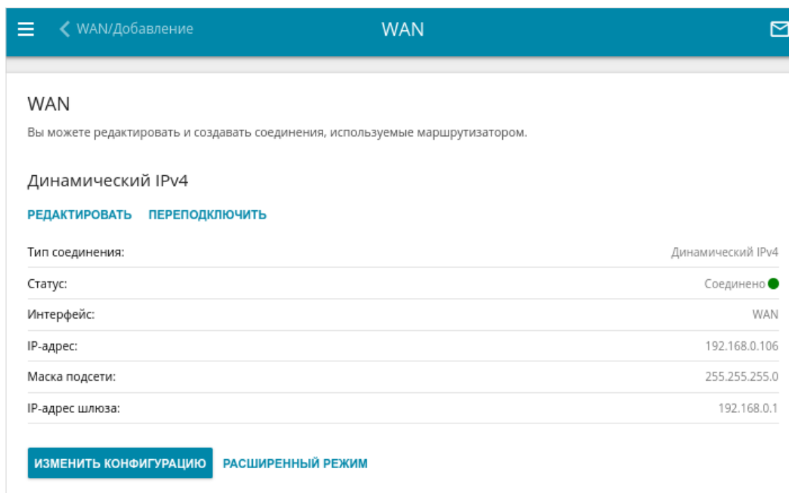
Рисунок 69. Страница Настройка соединений / WAN . Упрощенный режим.
