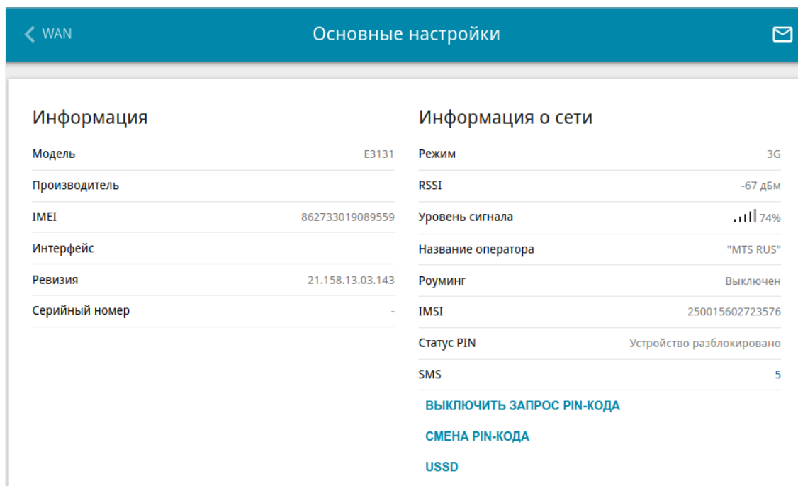
Рисунок 169. Страница USB-модем / Название модема / Основные настройки .
