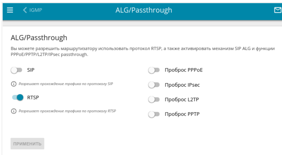
Рисунок 197. Страница Дополнительно / ALG/Passthrough .
