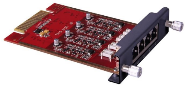
4FXO
