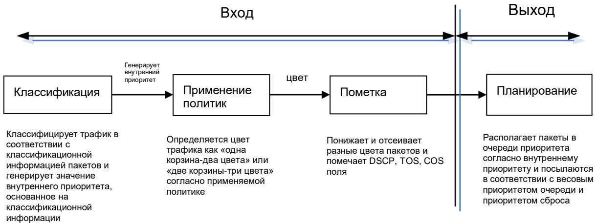
Рисунок 13. Базовая модель QoS
