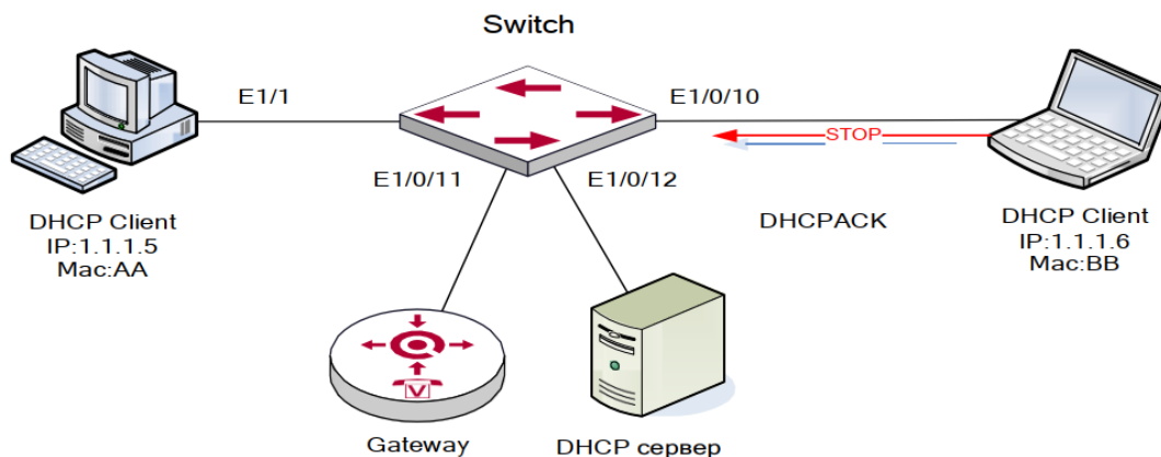
Рисунок 17. Типовое применение
