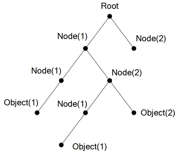
Рисунок 1. Пример дерева ASN.1
