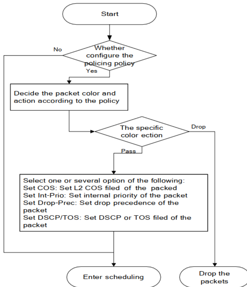
Рисунок 15. Процессы регулирования и пометки
