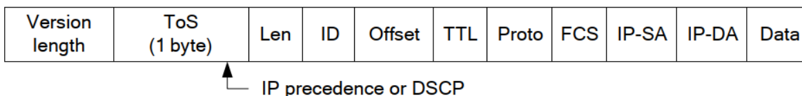
Рисунок 11. Приоритет ToS
