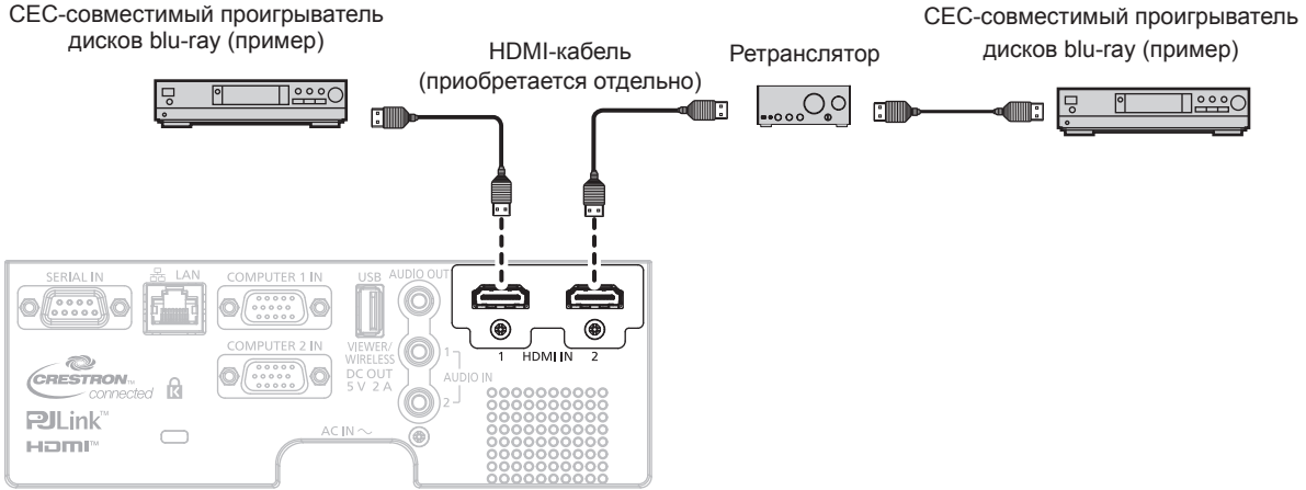
Пример подключения с CEC-совместимым устройством
