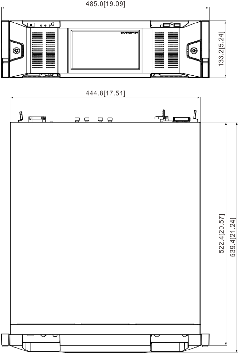
Рис. 2-4 Габариты панели с дисплеем (мм[дюймы])
