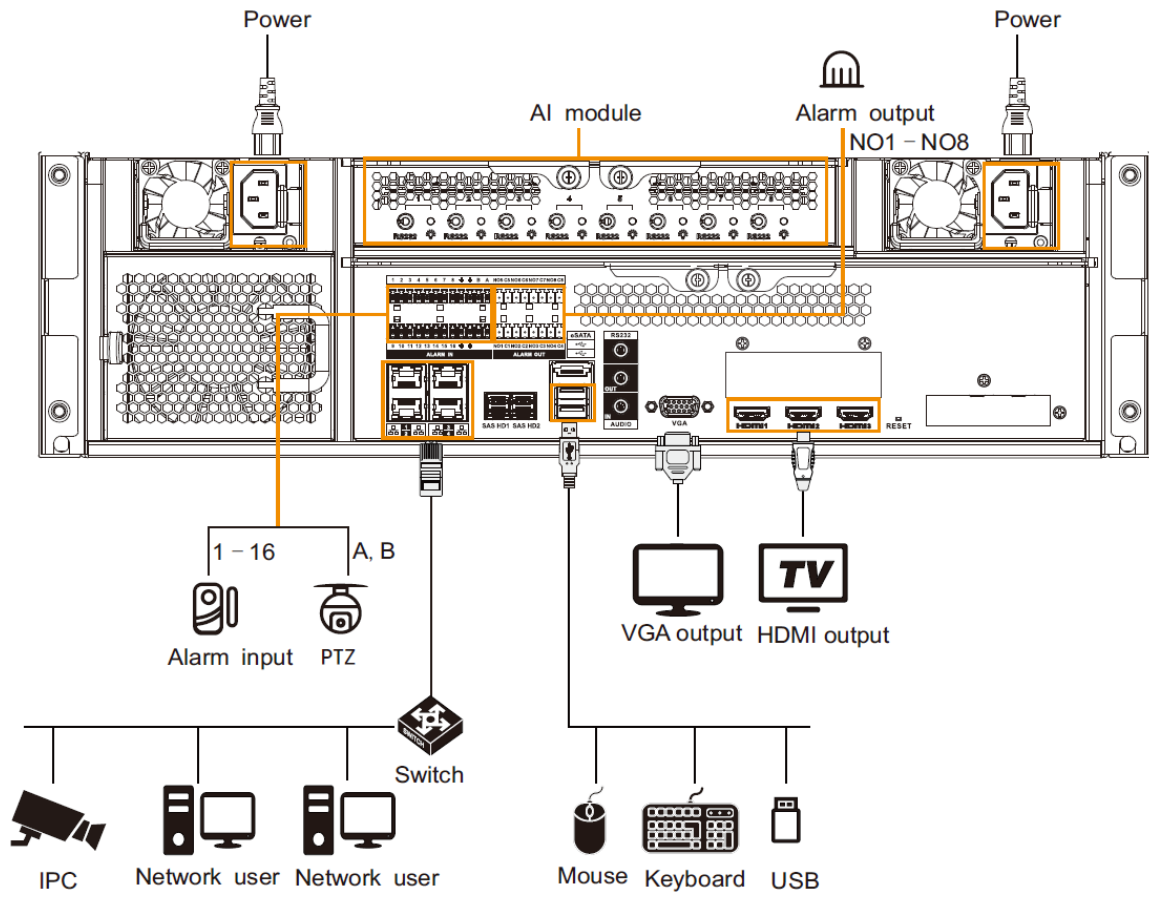
Рис. 3-2 Схема подключения
