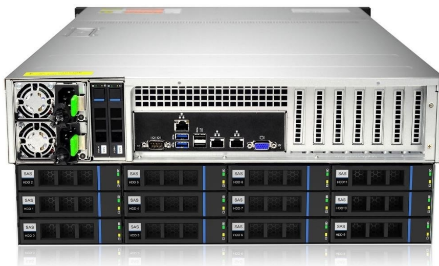
Рисунок 2. Серверная платформа QSRV-VS-463602RMC (Вид сзади)
