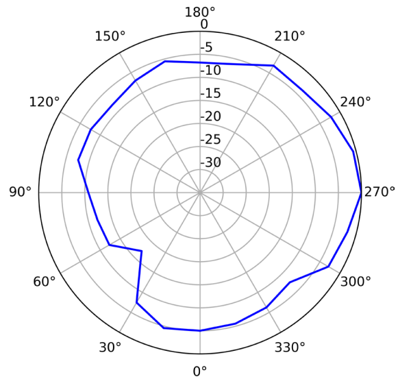
5G (Vertical)
