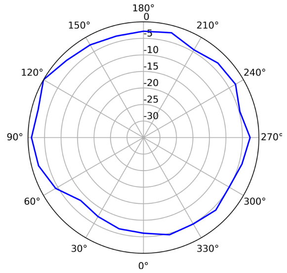
2.4G (Vertical)
