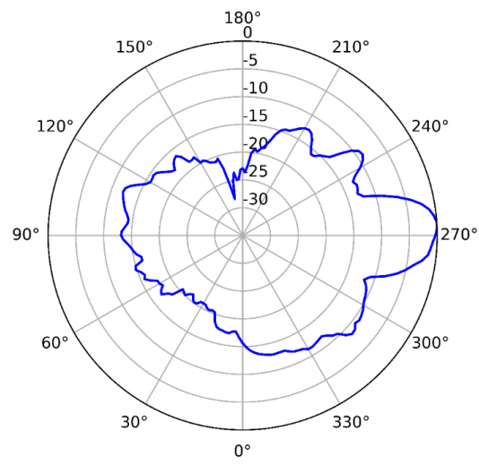
5GHz (Vertical)
