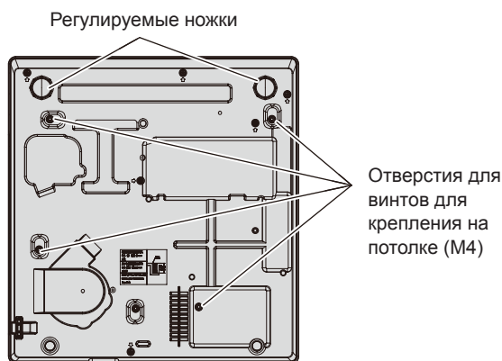
Положения отверстий для винтов для крепления на потолке и регулируемых ножек
