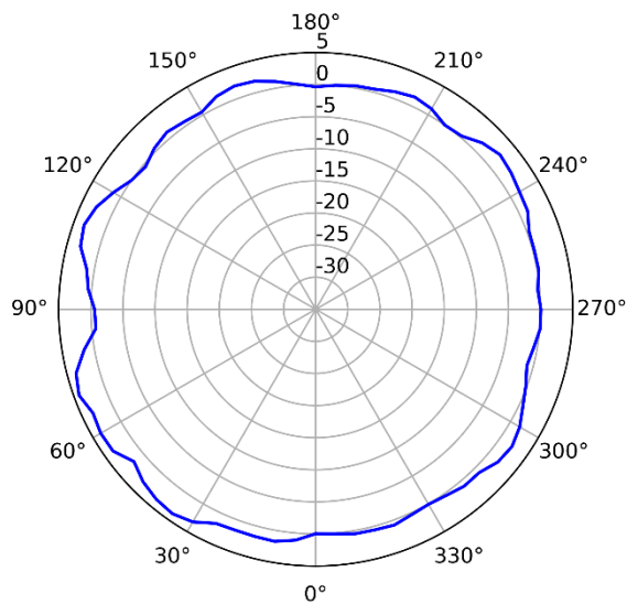
5GHz (Horizontal)
