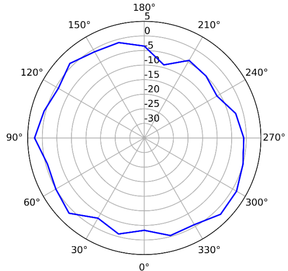
5GHz (Vertical)
