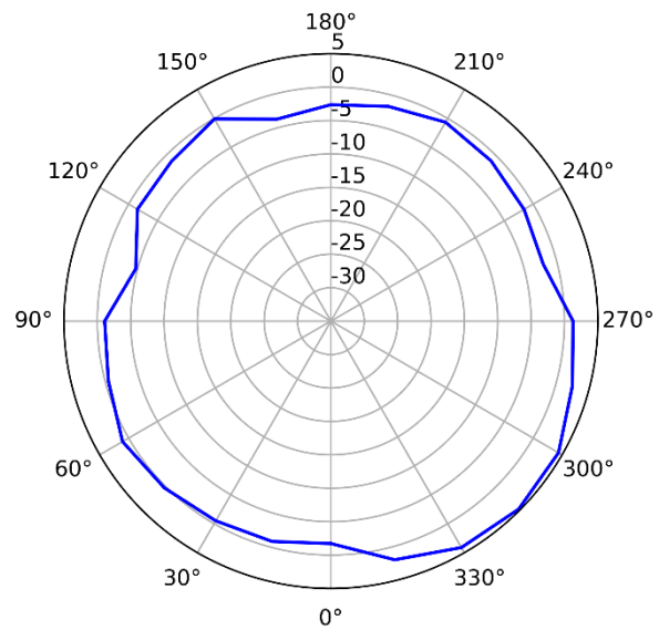
2.4GHz (Vertical)
