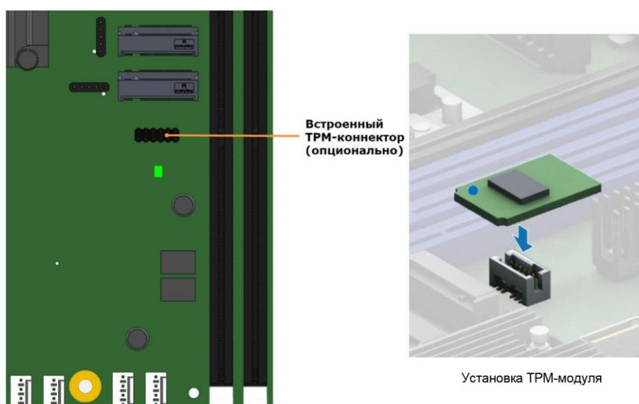
Рисунок 82. Встроенный разъем TPM
