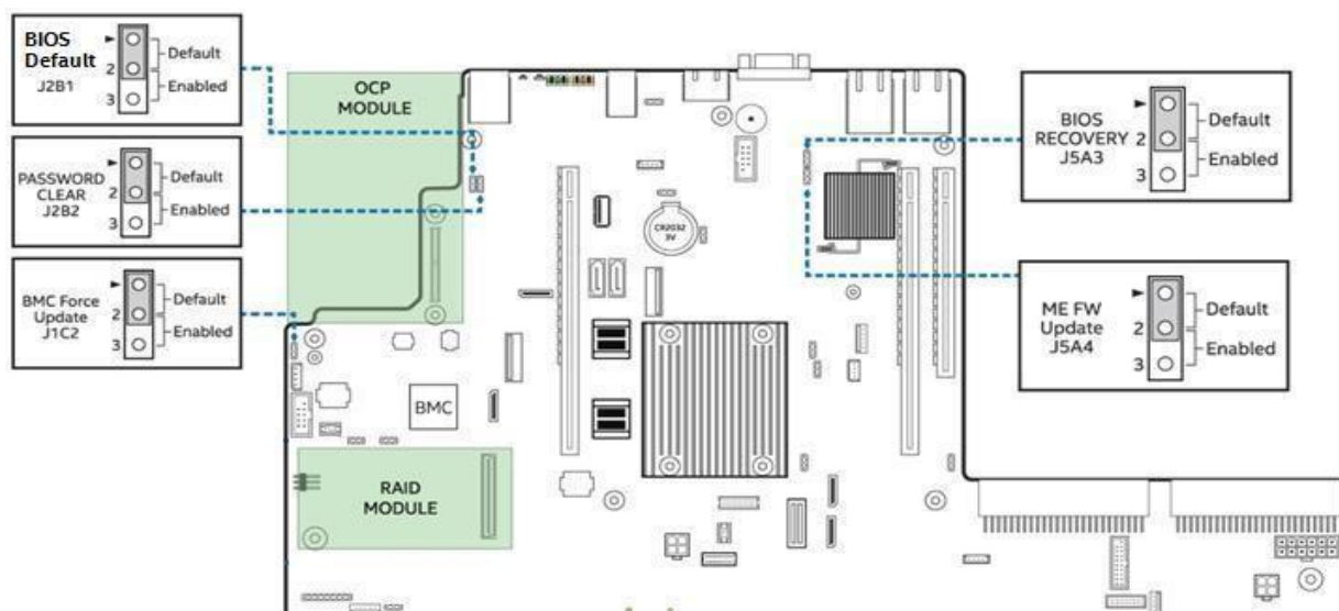
Рисунок 14. Переключатели для настройки платы
