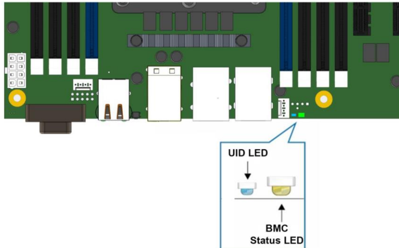
Рисунок 85. Светодиодный индикатор состояния системы и идентификационный светодиодный индикатор
