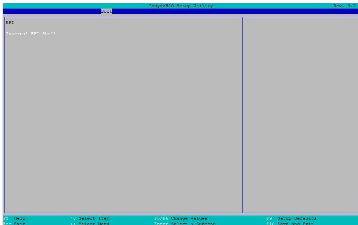
Рисунок 132. Меню EFI
