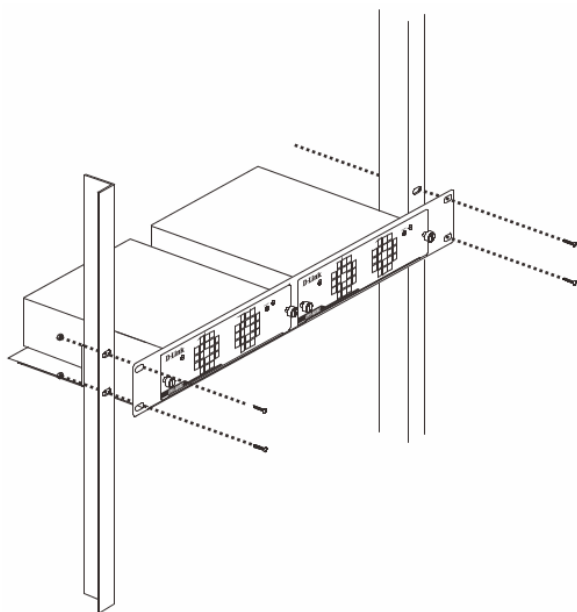
Рисунок 12 — Установка DPS-800 в стандартную стойку для оборудования
