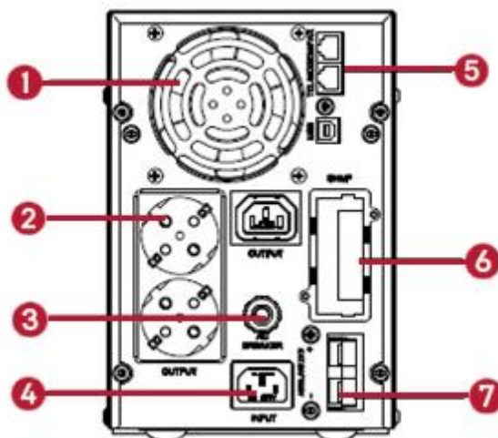
Рисунок 2. Вид задней панели ИБП
