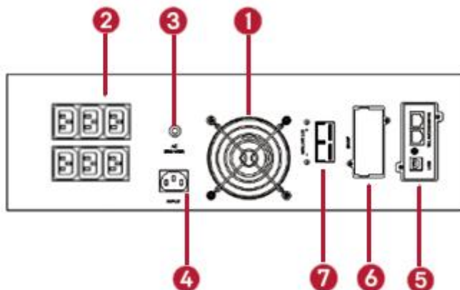
Рисунок 2. Вид задней панели 1500 и 3000 В·А
