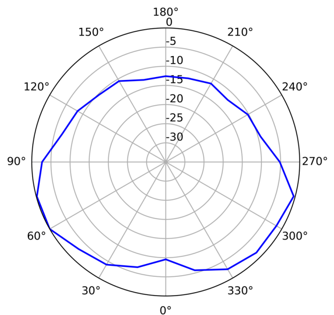
5GHz (Vertical)
