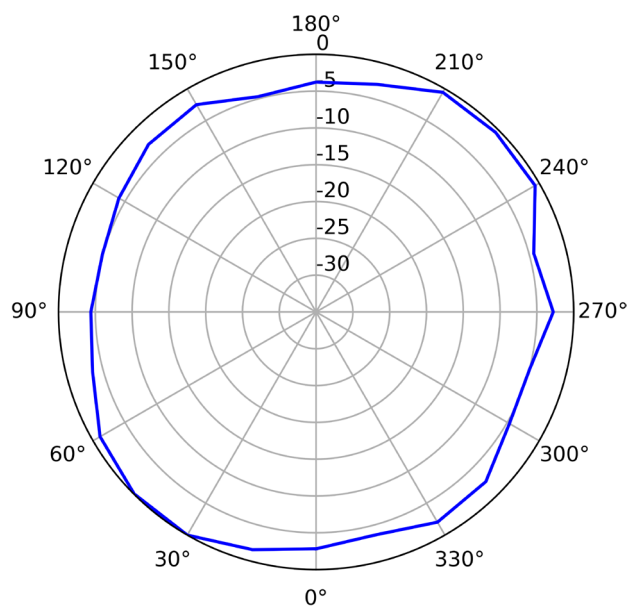
2.4G (Vertical)
