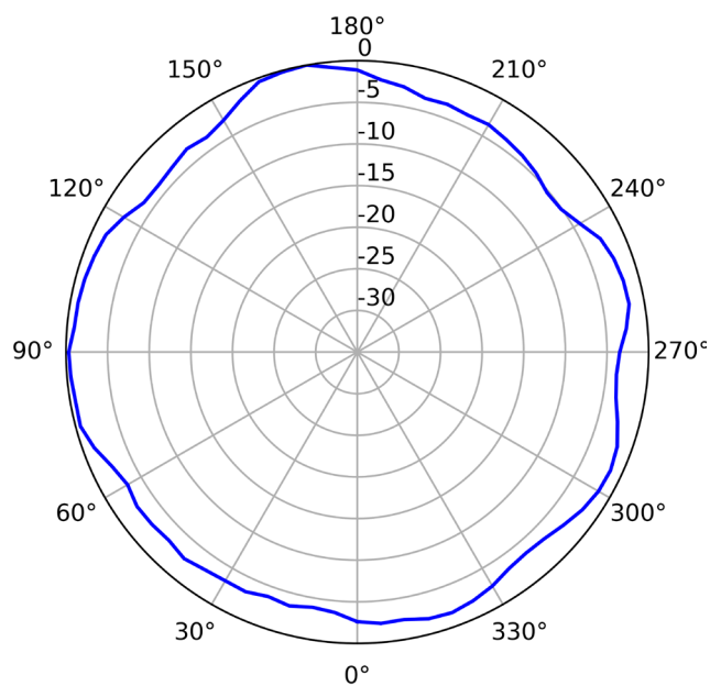
5G (Horizontal)
