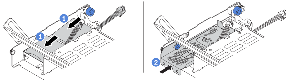
Рис. 168. Установка модуля суперконденсатора
