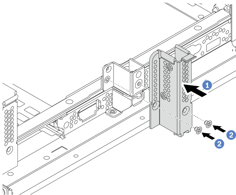
Рис. 176. Установка скобы задней стенки B1
