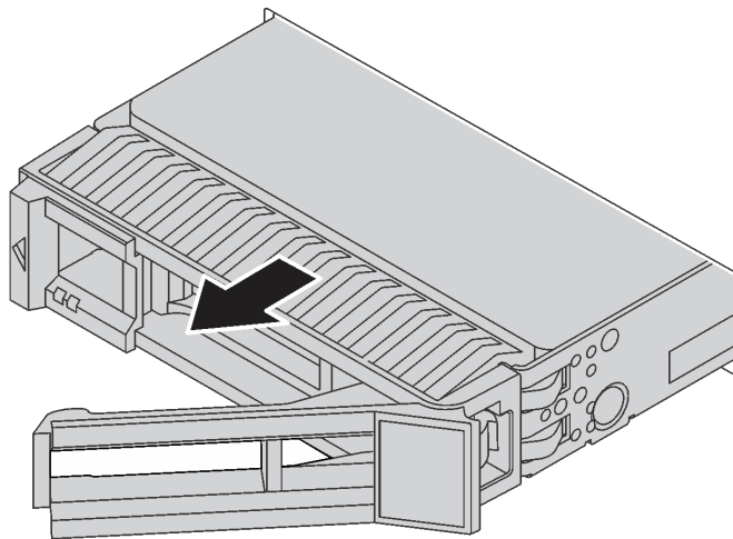
Рис. 77. Извлечение оперативно заменяемого диска
