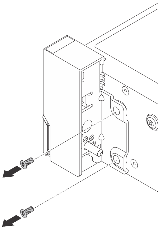
Рис. 152. Удаление винтов
