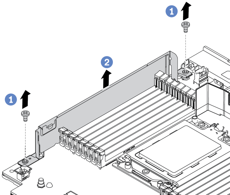
Рис. 57. Снятие держателей кабелей
