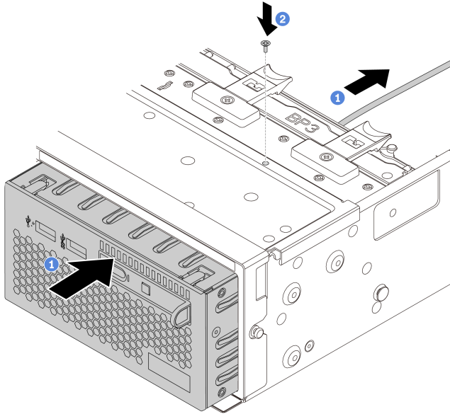
Рис. 66. Установка переднего блока ввода-вывода
