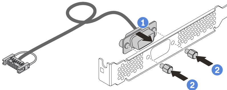
Рис. 196. Сборка модуля последовательного порта
