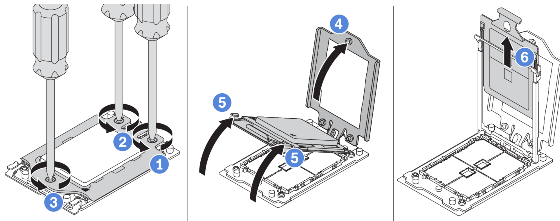
Рис. 212. Снятие процессора
