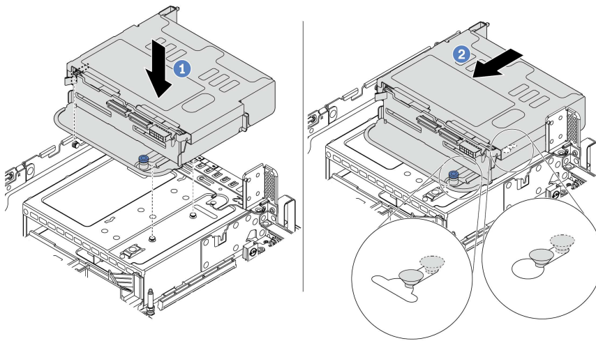
Рис. 112. Установка заднего отсека для четырех 2,5-дюймовых дисков
