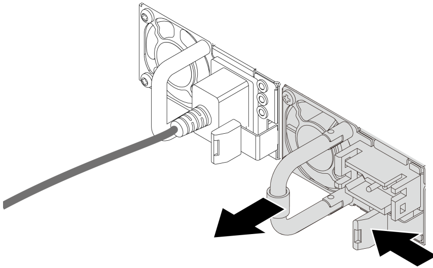
Рис. 124. Снятие оперативно заменяемого блока питания
