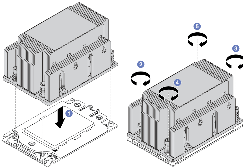
Рис. 215. Установка стандартного радиатора
