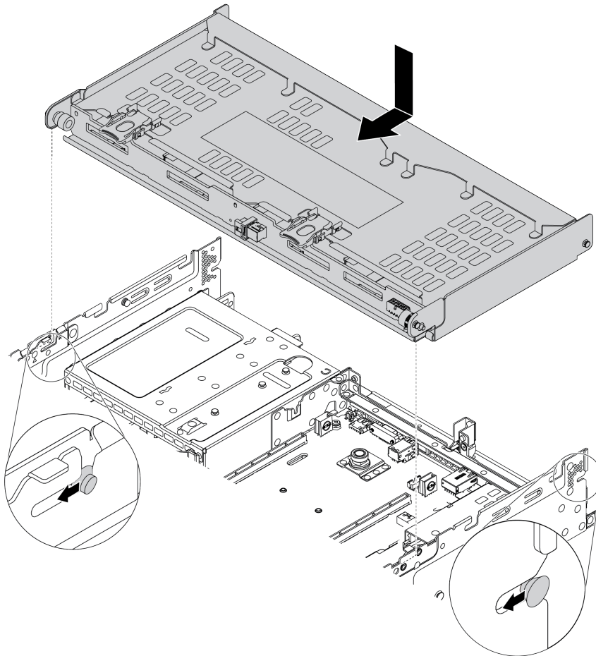
Рис. 109. Установка заднего отсека для четырех 3,5-дюймовых дисков
