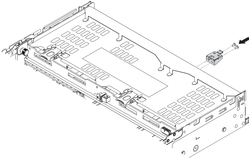
Рис. 110. Установка опорной скобы верхнего кожуха
