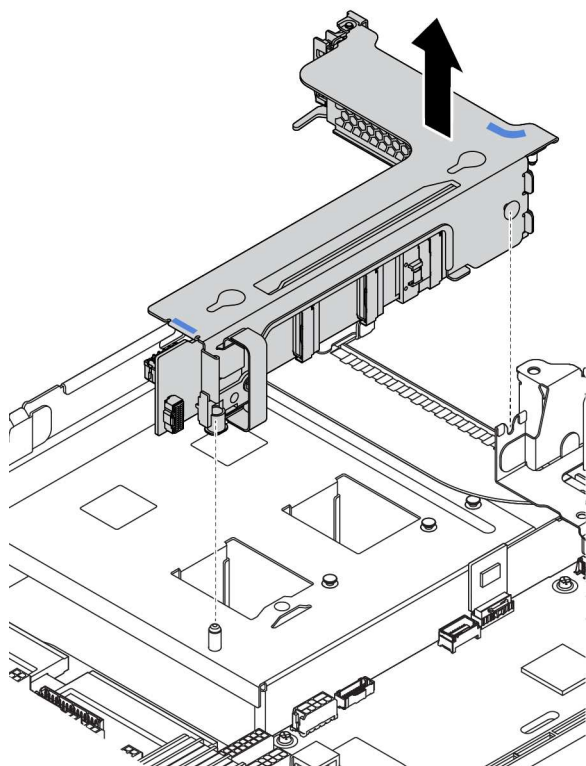
Рис. 189. Снятие блока платы-адаптера Riser 3 (скоба платы с двумя гнездами)
