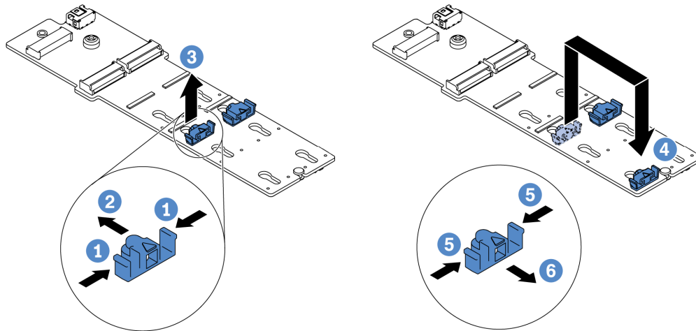
Рис. 138. Регулировка фиксатора M.2
