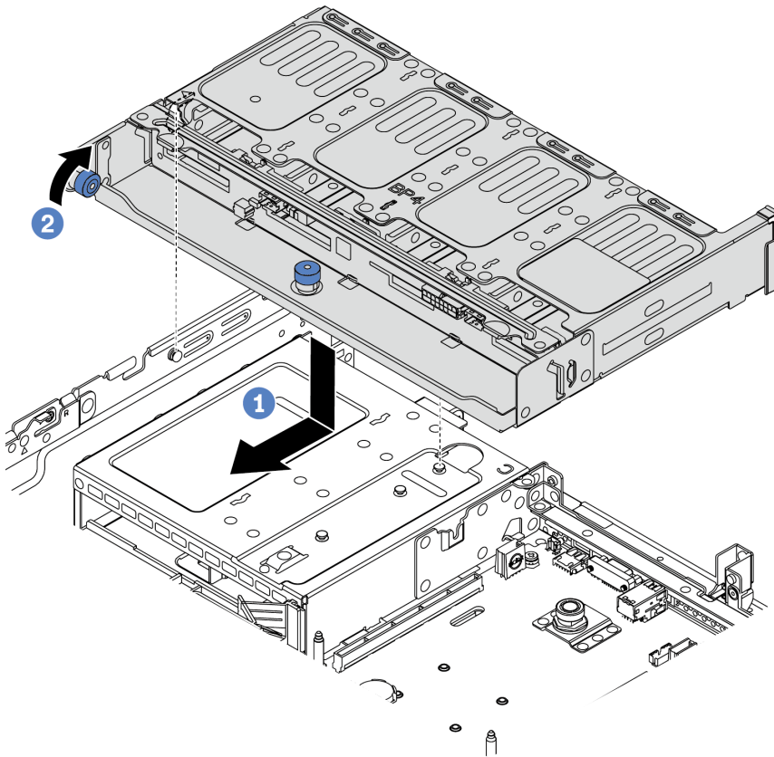
Рис. 114. Установка заднего отсека для восьми 2,5-дюймовых дисков
