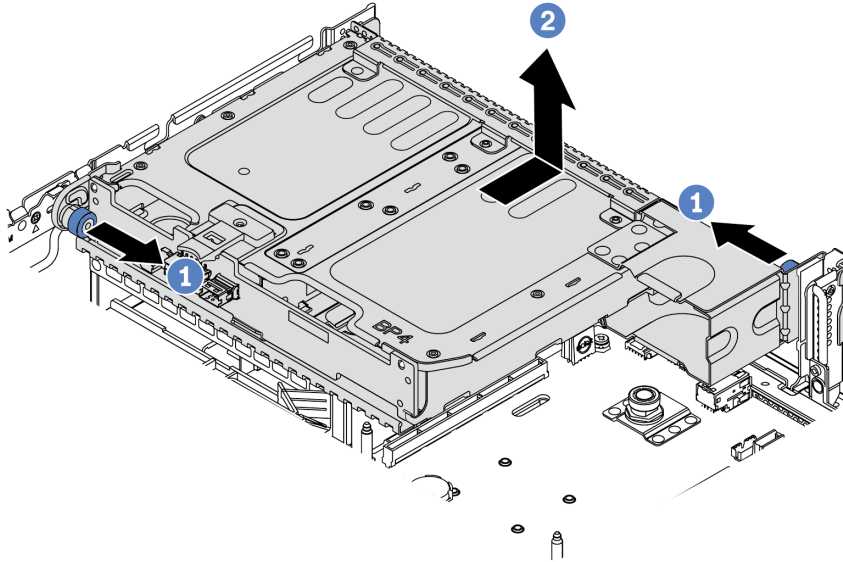
Рис. 106. Снятие заднего отсека для двух 3,5-дюймовых дисков
