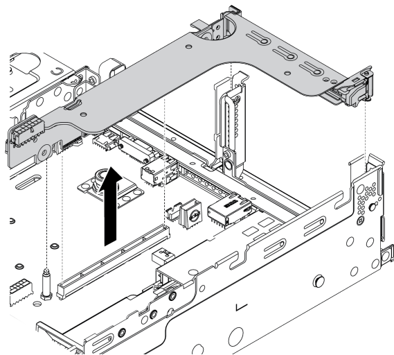
Рис. 180. Снятие блока платы-адаптера Riser 1/2 (скоба платы с одним гнездом)
