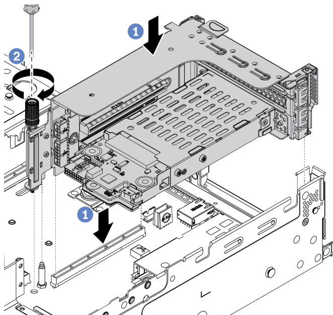
Рис. 121. Установка отсека для дисков 7 мм
