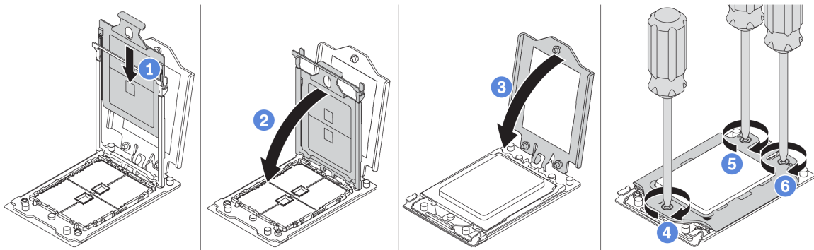
Рис. 213. Установка процессора
