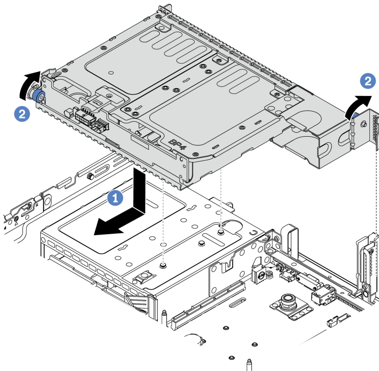
Рис. 107. Установка заднего отсека для двух 3,5-дюймовых дисков
