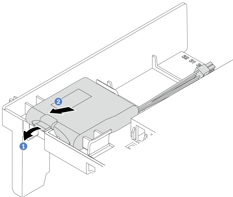
Рис. 162. Снятие модуля суперконденсатора
