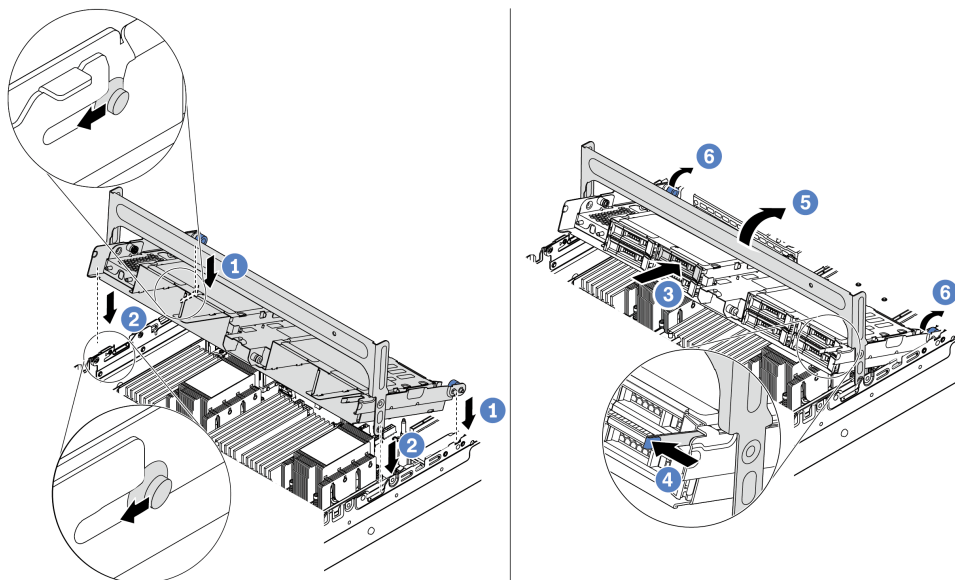
Рис. 100. Установка среднего отсека для 2,5-дюймовых дисков и самих дисков
