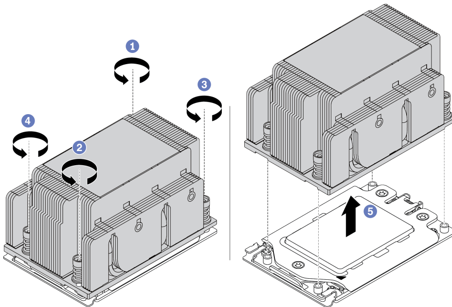
Рис. 210. Снятие стандартного радиатора
