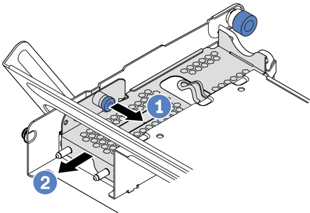
Рис. 167. Снятие металлического кожуха
