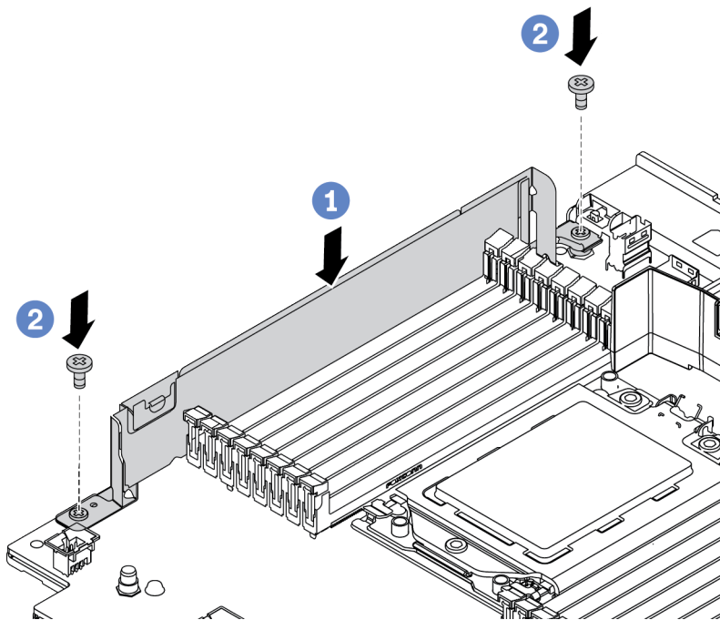
Рис. 58. Установка держателя кабеля
