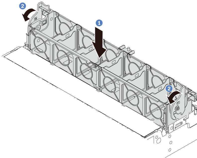
Рис. 205. Установка отсека вентиляторов компьютера
