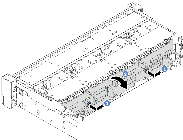
Рис. 86. Снятие объединительной панели для 3,5-дюймовых дисков
