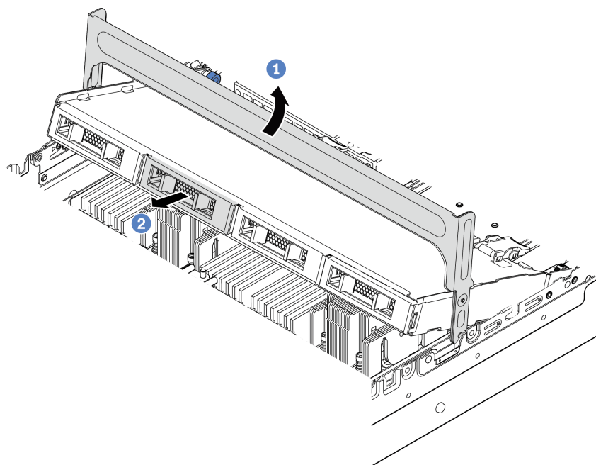
Рис. 101. Открытие ручки отсека для дисков и извлечение дисков
