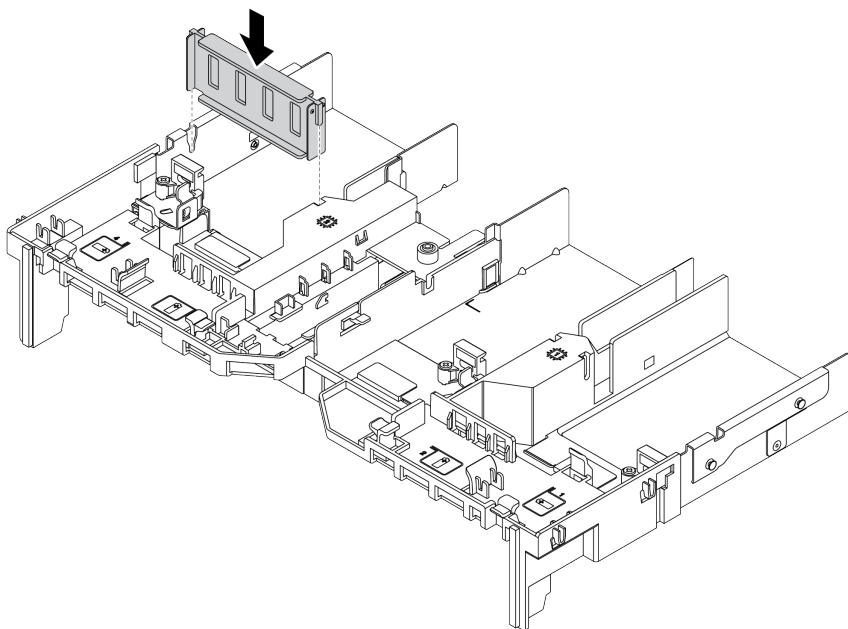
Рис. 75. Установка заглушки графического процессора
