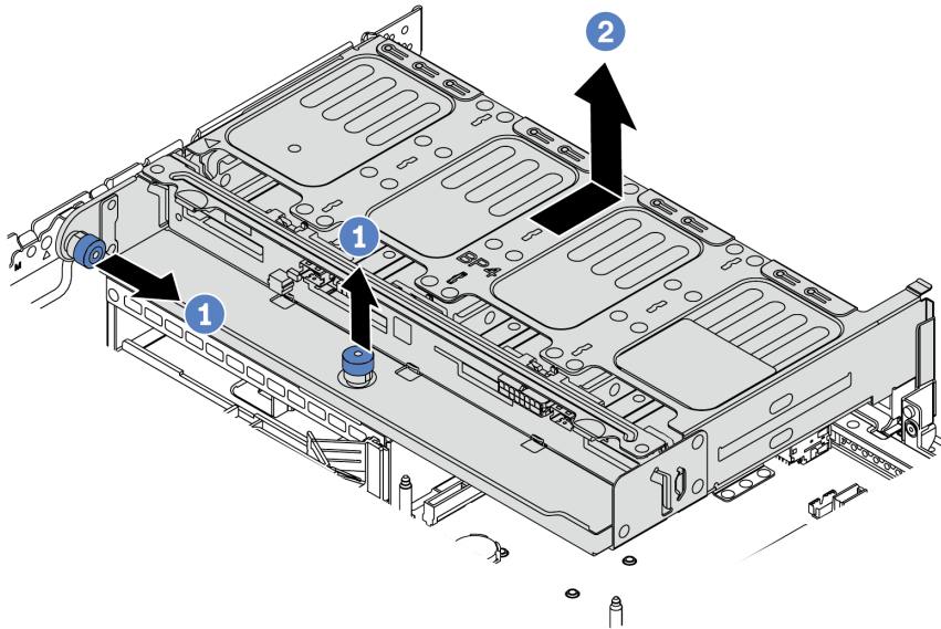
Рис. 113. Снятие заднего отсека для восьми 2,5-дюймовых дисков
