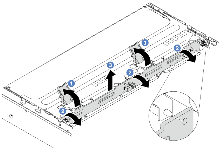
Рис. 89. Снятие объединительной панели для четырех 3,5-дюймовых дисков
