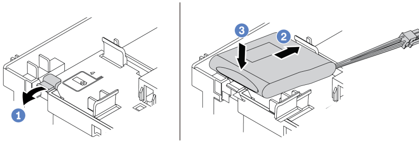
Рис. 163. Установка модуля суперконденсатора в дефлекторе
