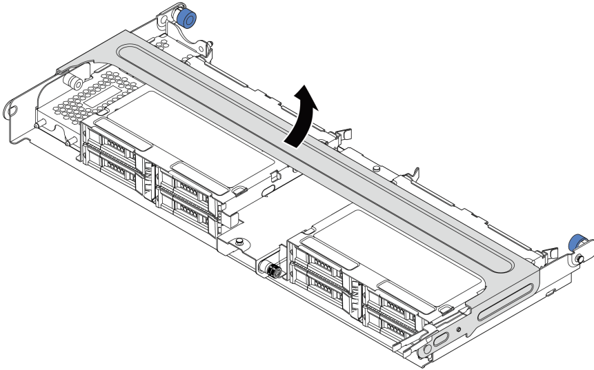
Рис. 166. Открытие ручки среднего отсека для диска
