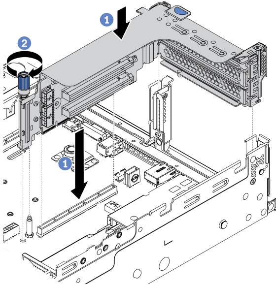
Рис. 187. Установка блока платы-адаптера Riser 1/2 (скоба платы с тремя гнездами)
