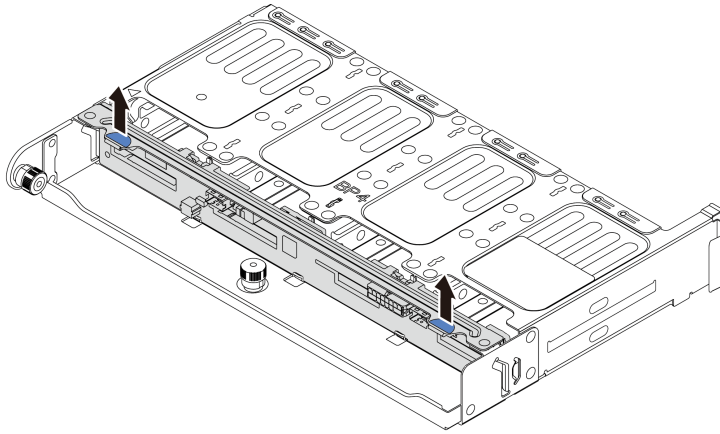
Рис. 83. Снятие объединительной панели для восьми 2,5-дюймовых дисков
