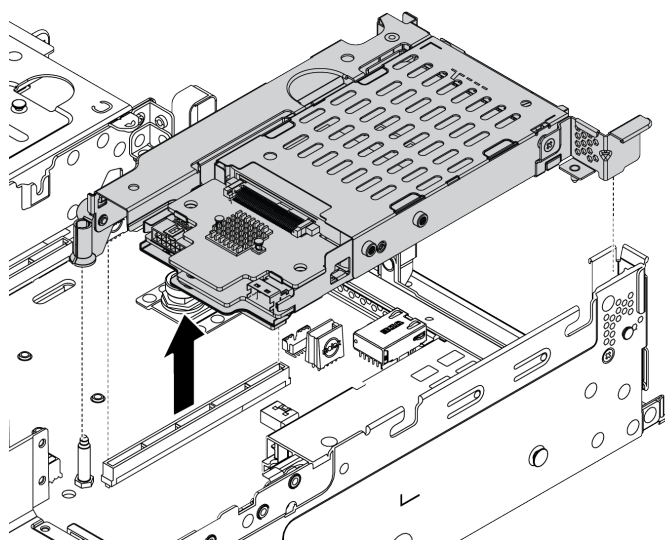
Рис. 118. Снятие блока платы-адаптера Riser
