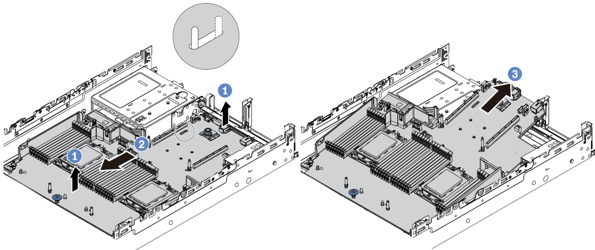
Рис. 217. Снятие материнской платы
