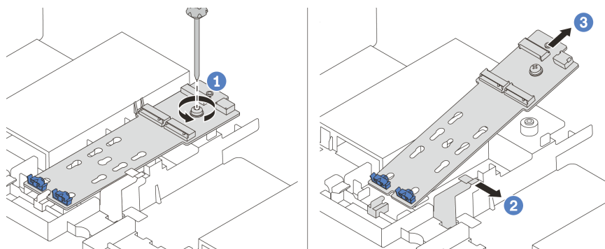
Рис. 137. Снятие адаптера M.2
