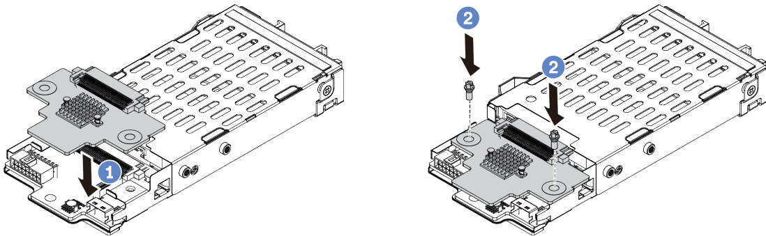
Рис. 95. Установка объединительной панели для дисков 7 мм (сверху)
