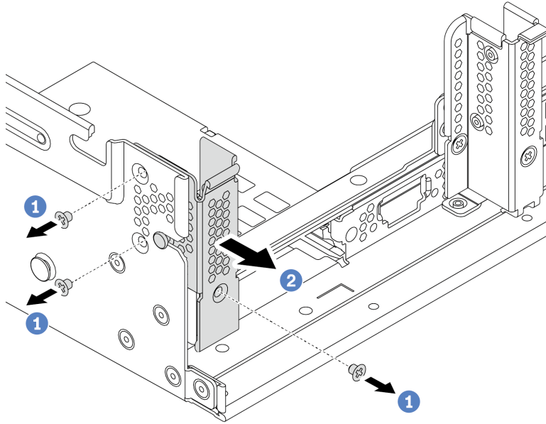
Рис. 173. Установка скобы задней стенки A1
