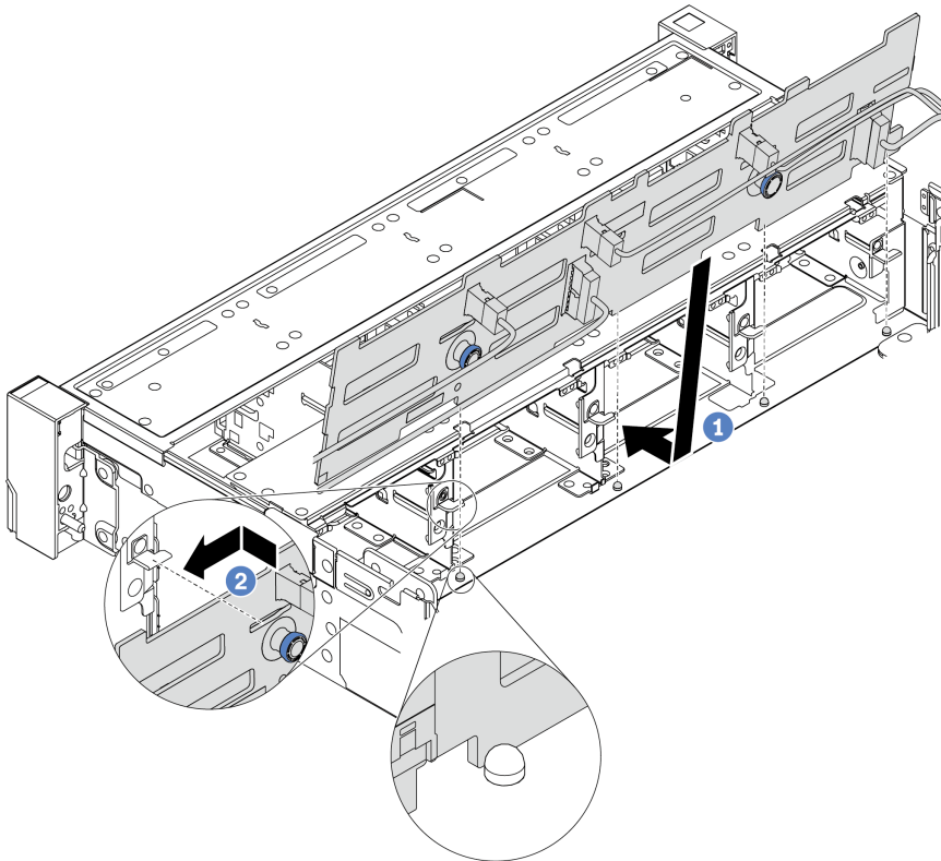
Рис. 87. Установка объединительной панели для 3,5-дюймовых дисков
