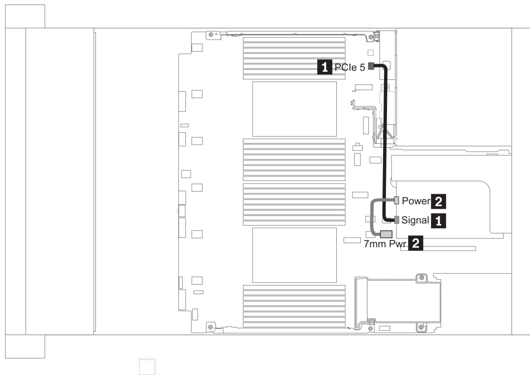
Рис. 19. 7mm cable routing
