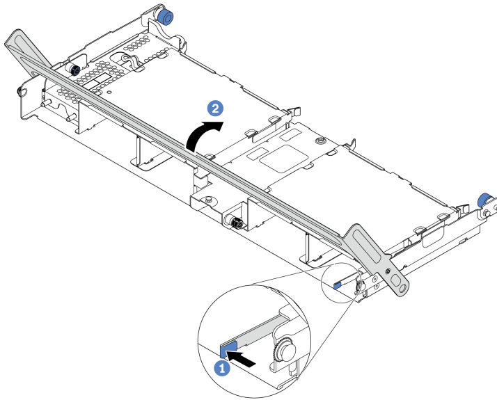
Рис. 98. Закрытие ручки среднего отсека для 2,5-дюймовых дисков
