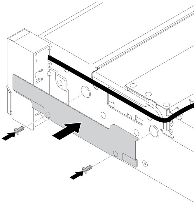
Рис. 156. Установка фиксатора кабелей
