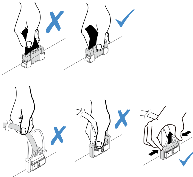
Рис. 63. Отключение кабелей переднего блока ввода-вывода
