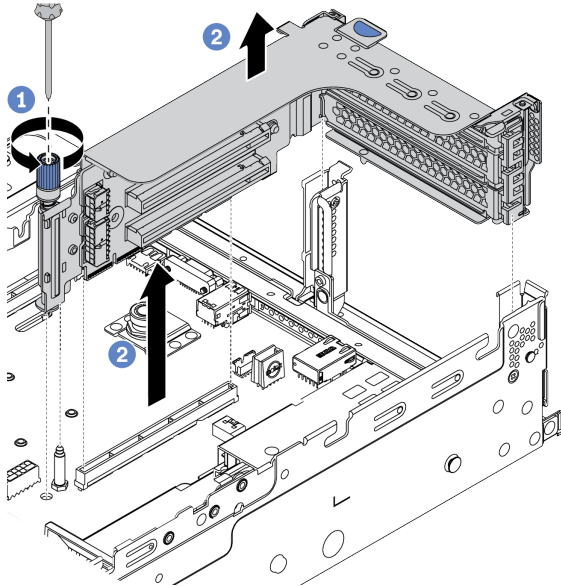
Рис. 179. Снятие блока платы-адаптера Riser 1/2 (скоба с тремя гнездами)
