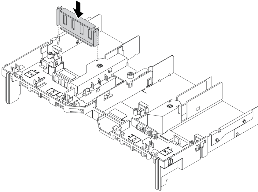
Рис. 71. Установка заглушки графического процессора
