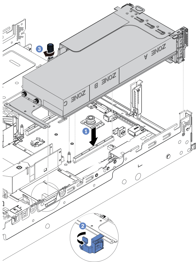
Рис. 74. Установка блока платы-адаптера Riser
