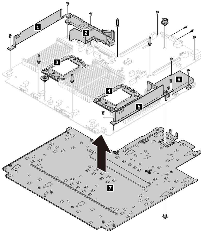
Рис. 220. Разборка материнской платы
