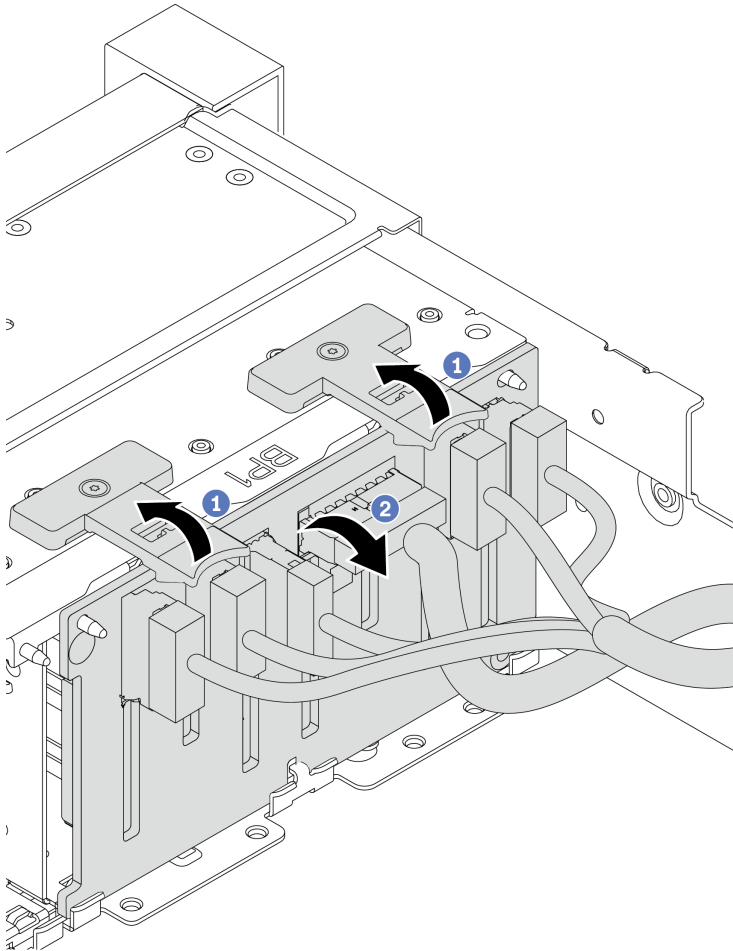
Рис. 80. Снятие объединительной панели для 2,5-дюймовых дисков
