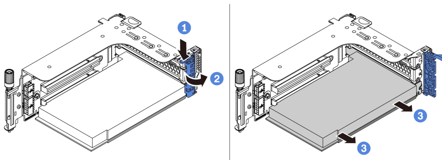
Рис. 190. Снятие адаптера PCIe
