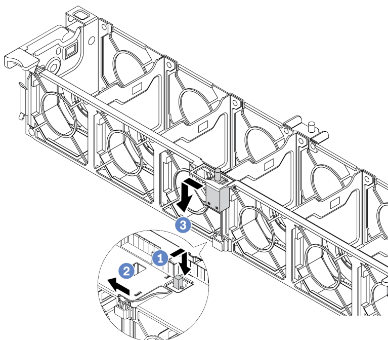
Рис. 130. Снятие датчика вмешательства
