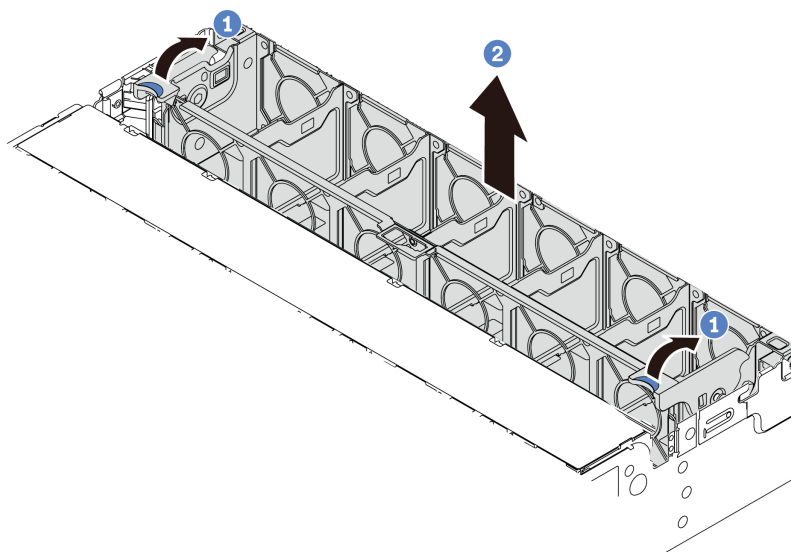
Рис. 204. Снятие отсека вентиляторов компьютера
