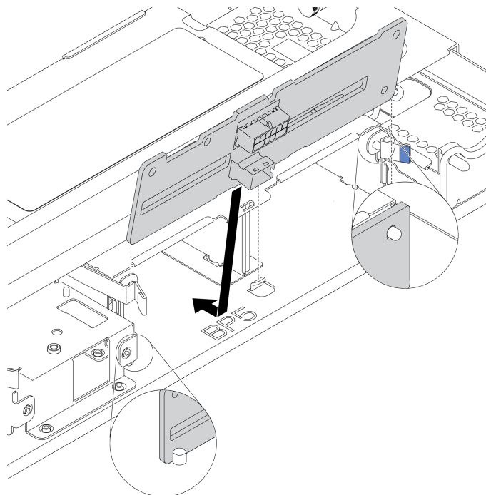
Рис. 99. Установка объединительной панели
