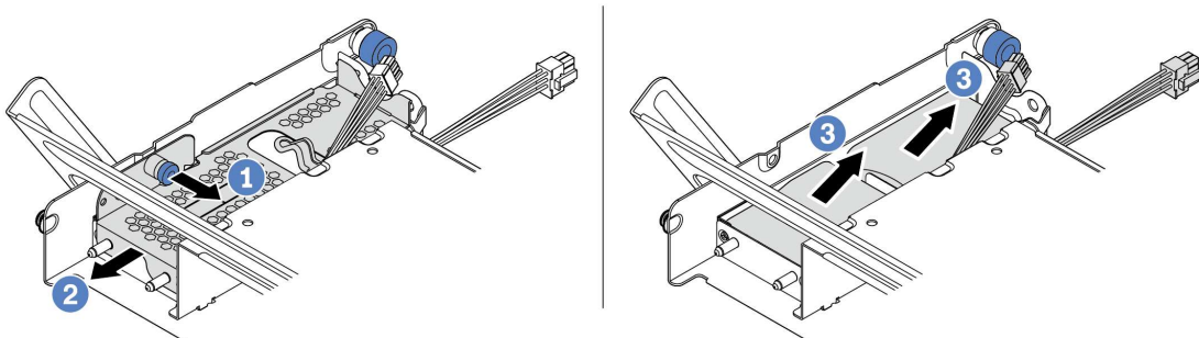
Рис. 165. Снятие модуля суперконденсатора
