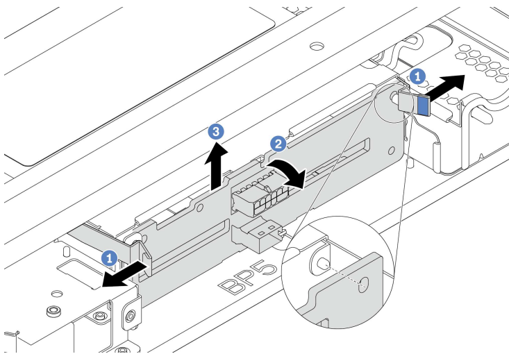
Рис. 82. Снятие объединительной панели для четырех 2,5-дюймовых дисков
