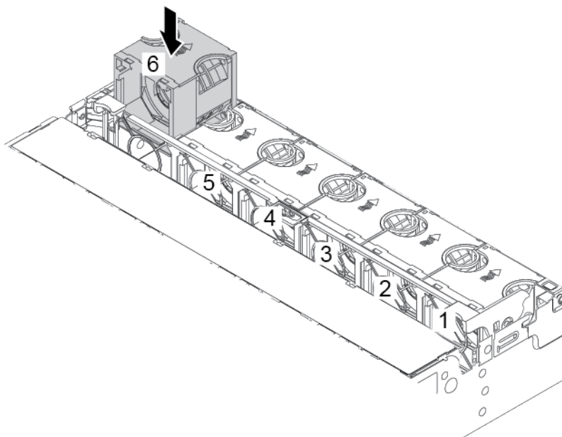
Рис. 203. Установка вентилятора компьютера
