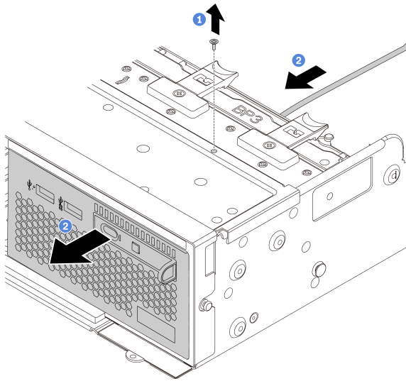
Рис. 64. Снятие переднего блока ввода-вывода
