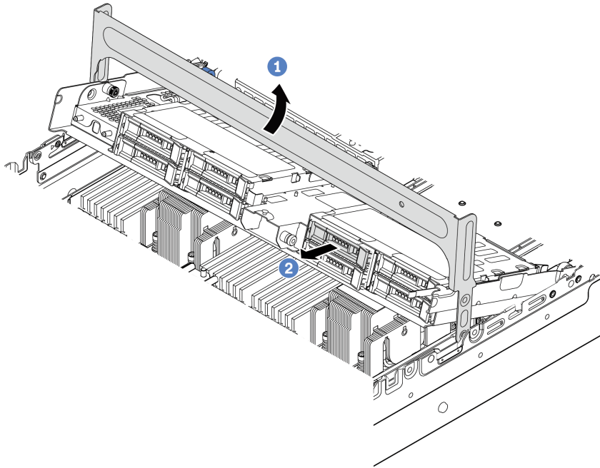
Рис. 96. Открытие ручки отсека для дисков и извлечение дисков
