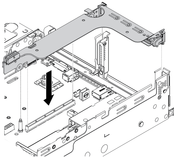
Рис. 188. Установка блока платы-адаптера Riser 1/2 (скоба платы с одним гнездом)
