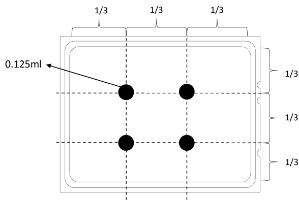
Рис. 214. Нанесение термопасты
