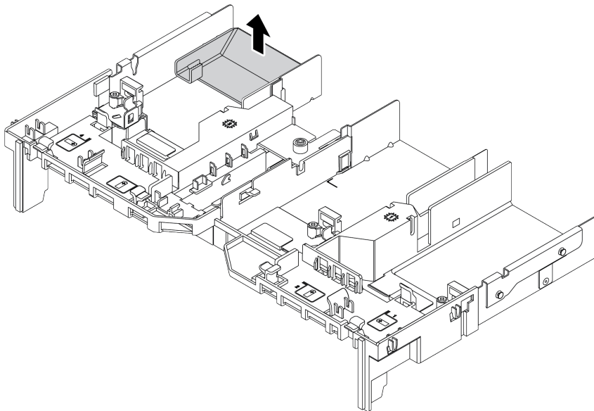
Рис. 70. Снятие дополнительного дефлектора
