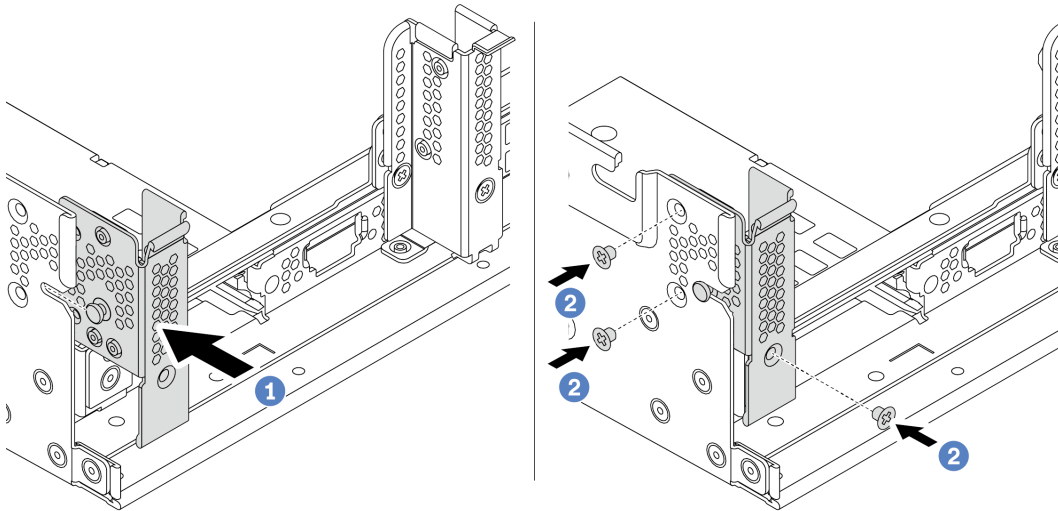
Рис. 174. Установка скобы задней стенки A1
