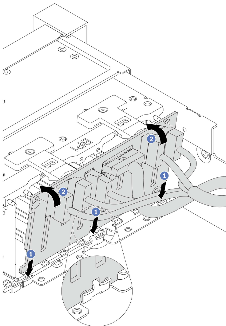
Рис. 81. Установка объединительной панели для 2,5-дюймовых дисков
