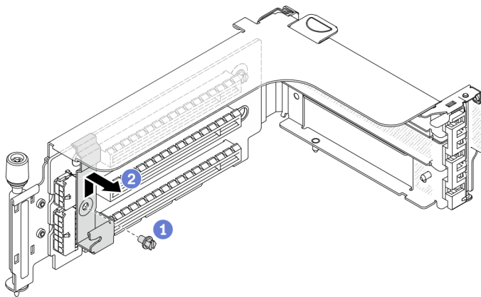
Рис. 117. Снятие фиксатора с отсека для дисков 7 мм
