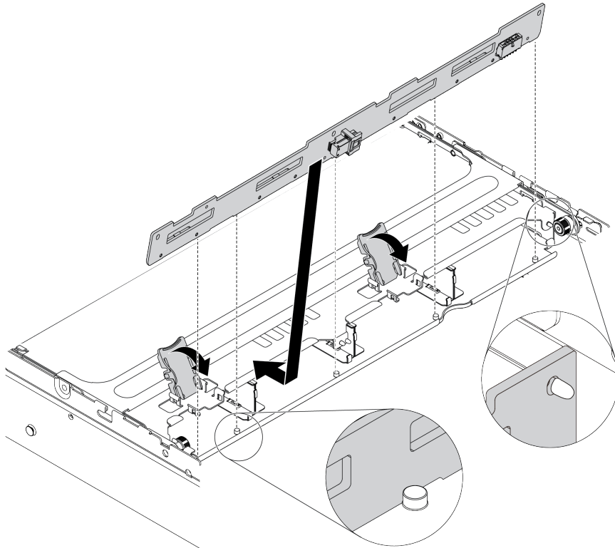
Рис. 91. Установка объединительной панели для четырех 3,5-дюймовых дисков
