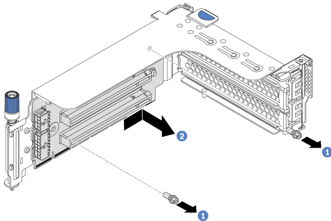
Рис. 182. Снятие платы-адаптера Riser (скоба с тремя гнездами)
