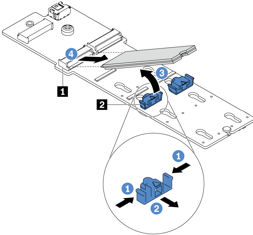
Рис. 136. Снятие диска M.2
