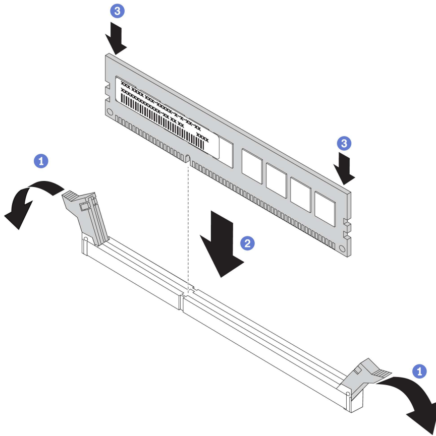
Рис. 144. Установка модуля памяти
