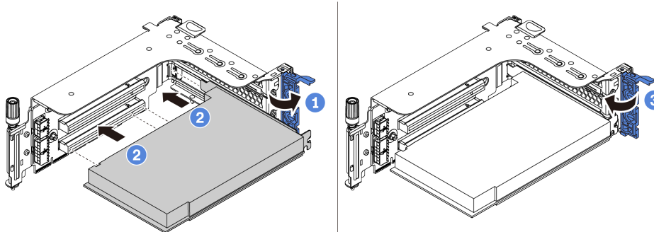
Рис. 186. Установка адаптера PCIe
