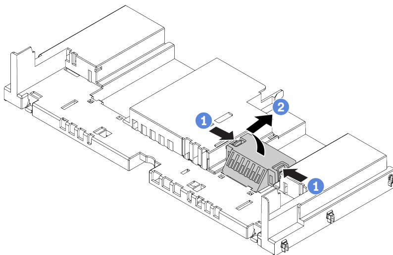
Рис. 54. Снятие заглушек со стандартного дефлектора
