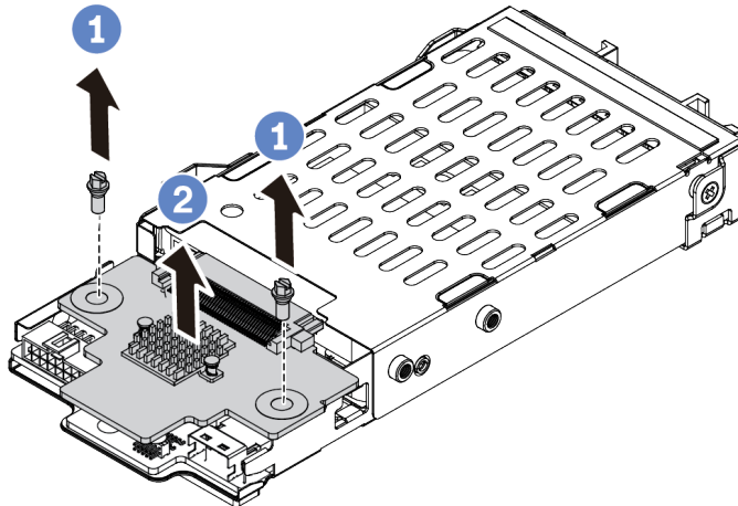
Рис. 92. Снятие объединительной панели для дисков 7 мм (сверху)
