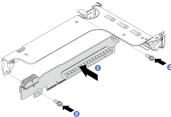
Рис. 185. Установка платы-адаптера Riser (скоба платы с одним или двумя гнездами)
