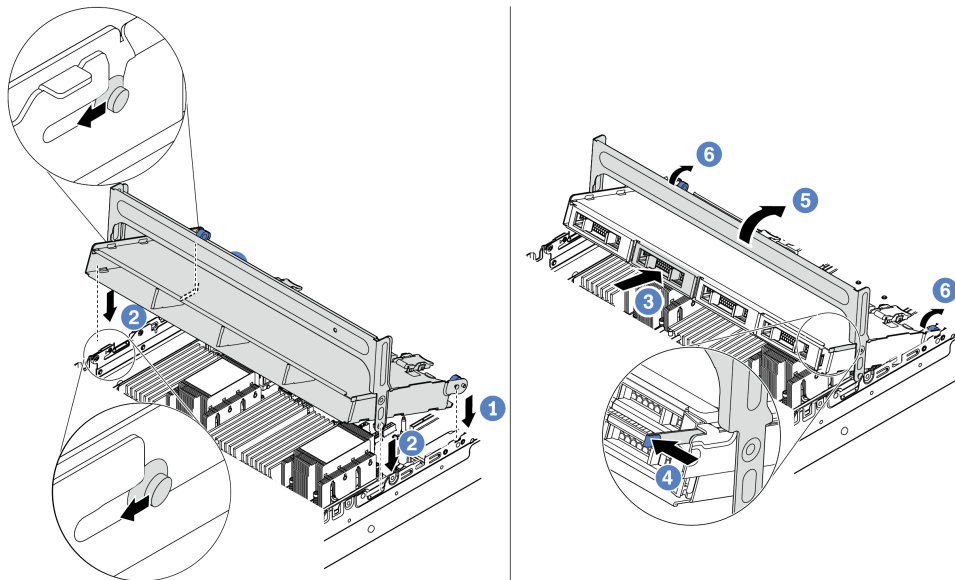
Рис. 105. Установка среднего отсека для 3,5-дюймовых дисков и самих дисков
