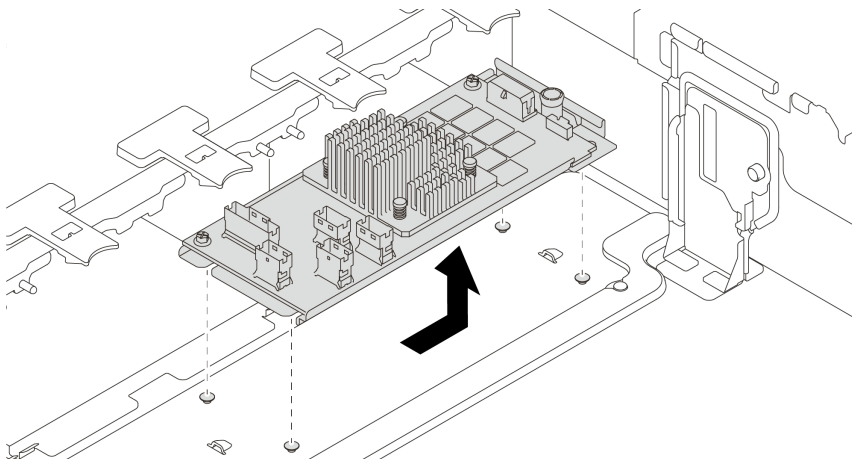
Рис. 128. Снятие внутреннего адаптера RAID/HBA/расширителя RAID CFF
