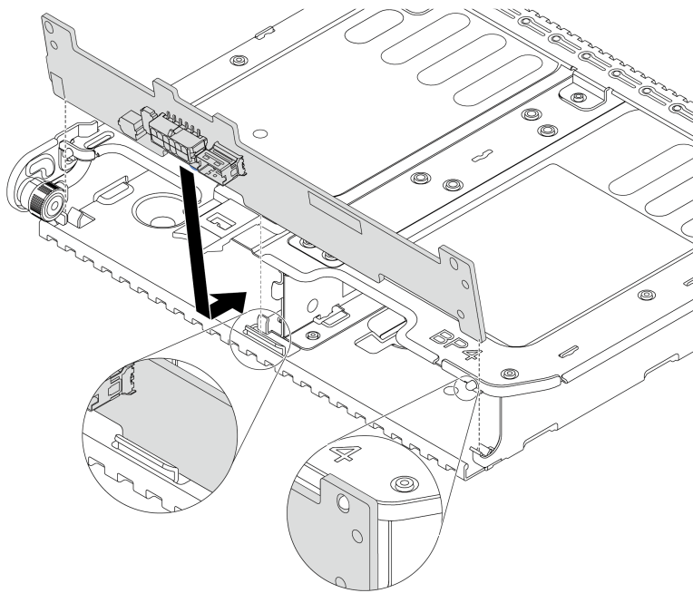
Рис. 90. Установка объединительной панели для двух 3,5-дюймовых дисков
