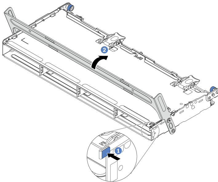
Рис. 103. Закрытие ручки среднего отсека для 3,5-дюймовых дисков
