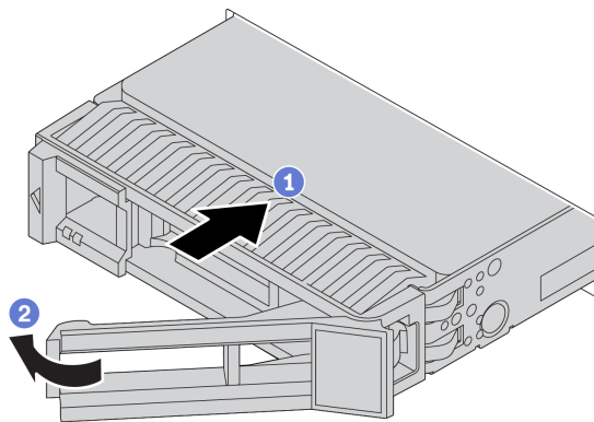
Рис. 79. Установка оперативно заменяемого диска
