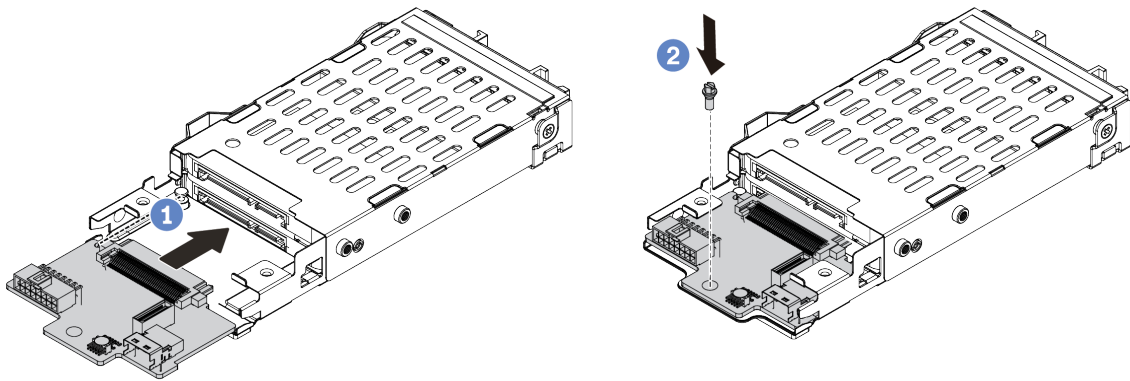
Рис. 94. Установка объединительной панели для дисков 7 мм (снизу)
