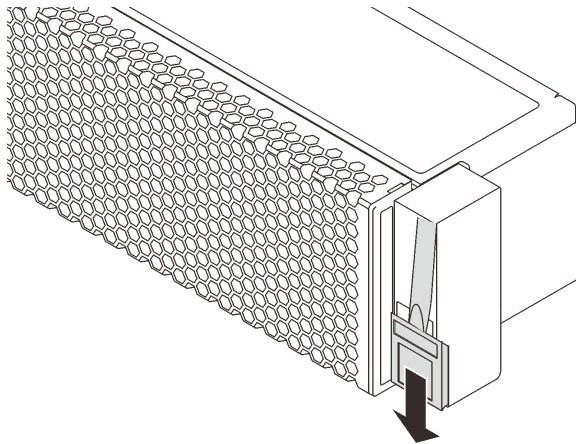
Рис. 149. Снятие пластинки с идентификационной этикеткой
