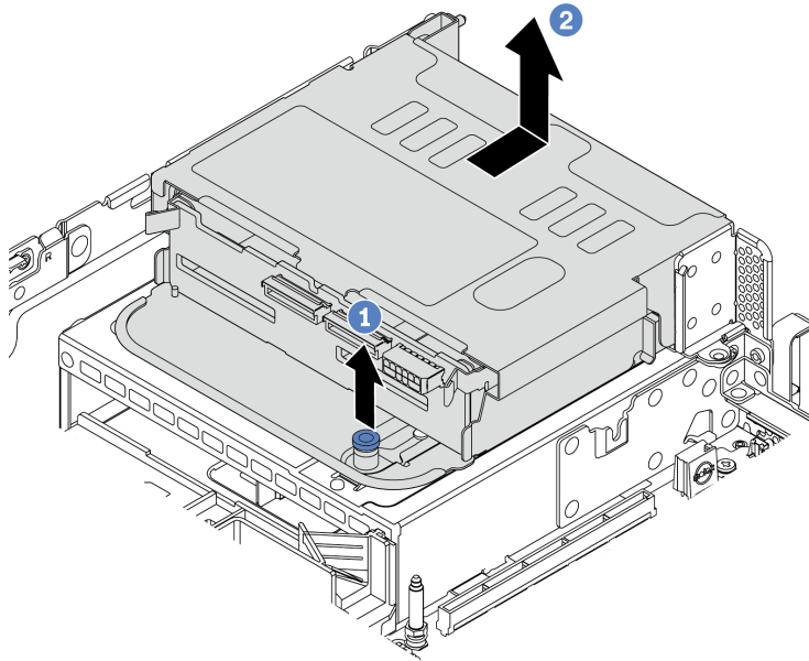
Рис. 111. Снятие заднего отсека для четырех 2,5-дюймовых дисков
