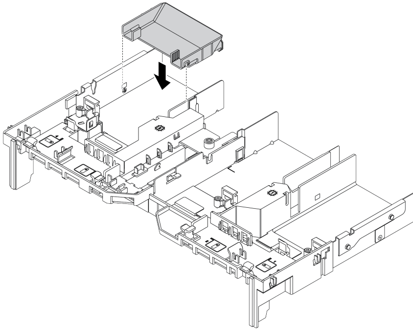
Рис. 72. Установка дополнительного дефлектора графического процессора
