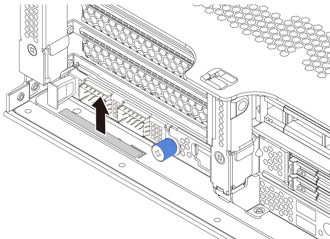
Рис. 146. Снятие этикетки OCP
