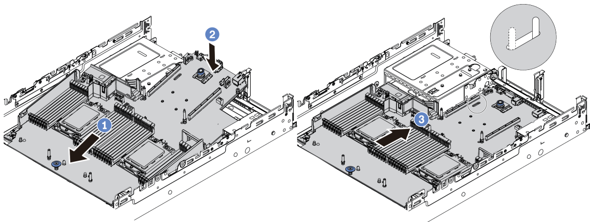
Рис. 218. Установка материнской платы
