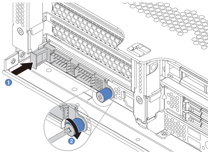
Рис. 147. Установка адаптера Ethernet OCP 3.0
