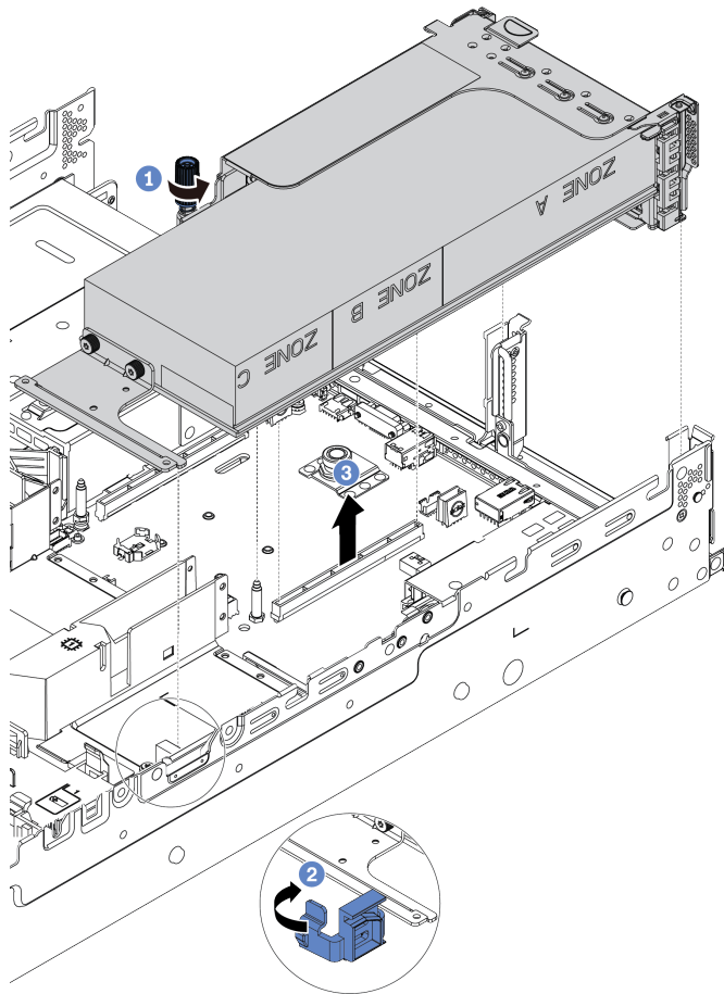
Рис. 68. Снятие блока платы-адаптера Riser
