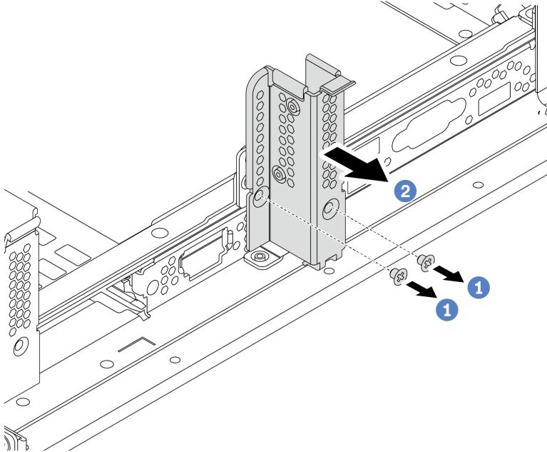
Рис. 175. Снятие скобы задней стенки B1
