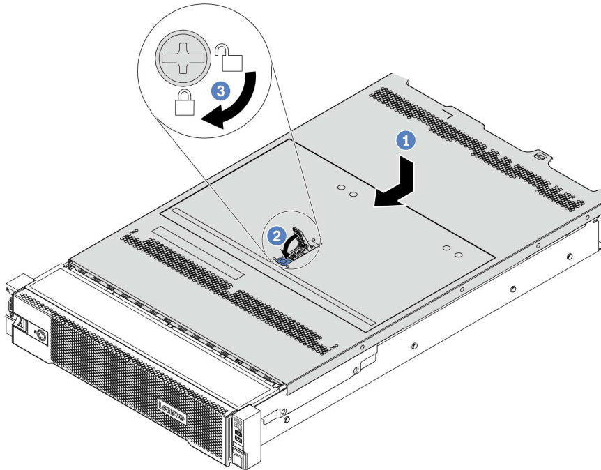
Рис. 209. Установка верхнего кожуха
