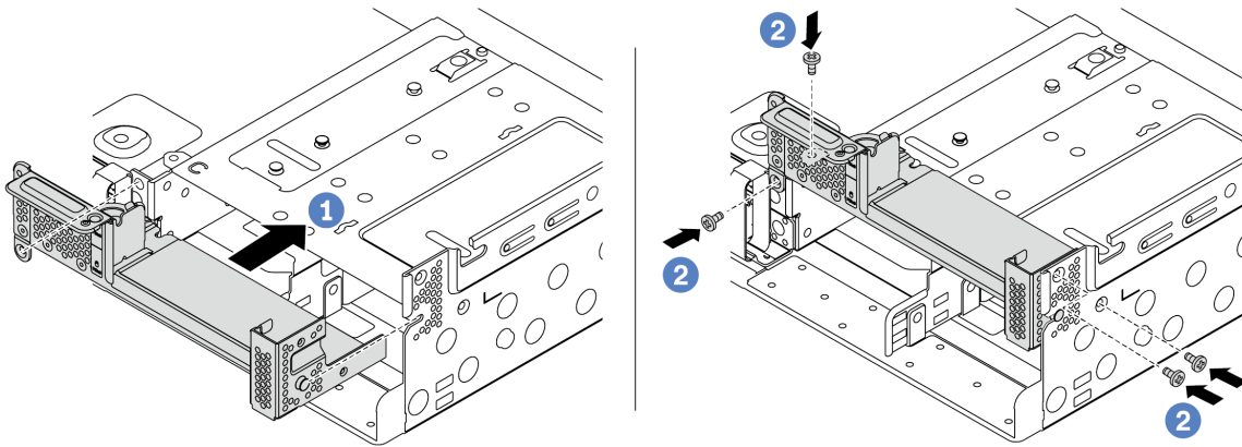
Рис. 178. Установка скобы задней стенки C1
