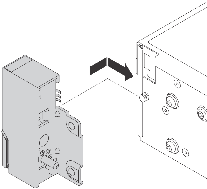
Рис. 154. Установка защелки стойки
