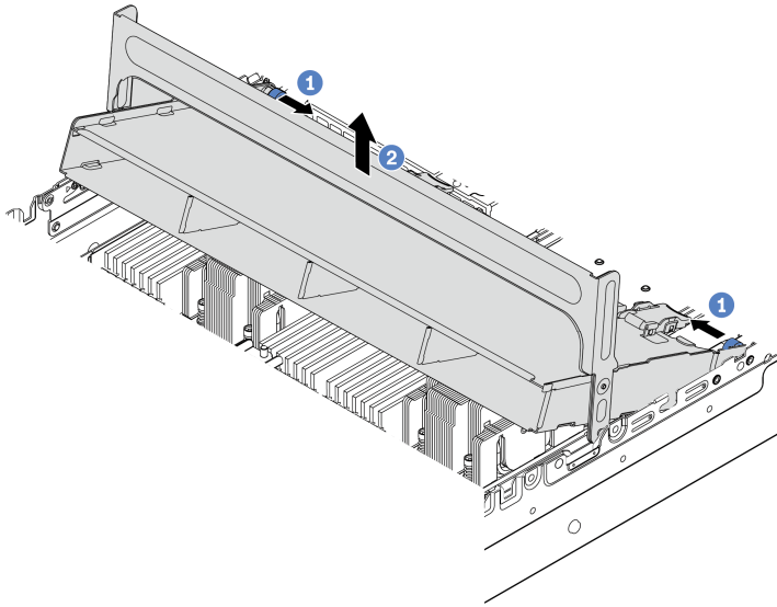
Рис. 102. Снятие среднего отсека для 3,5-дюймовых дисков
