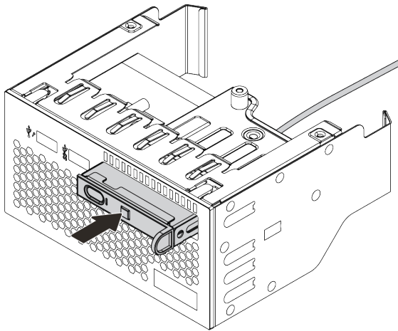
Рис. 67. Установка ЖК-панели диагностики
