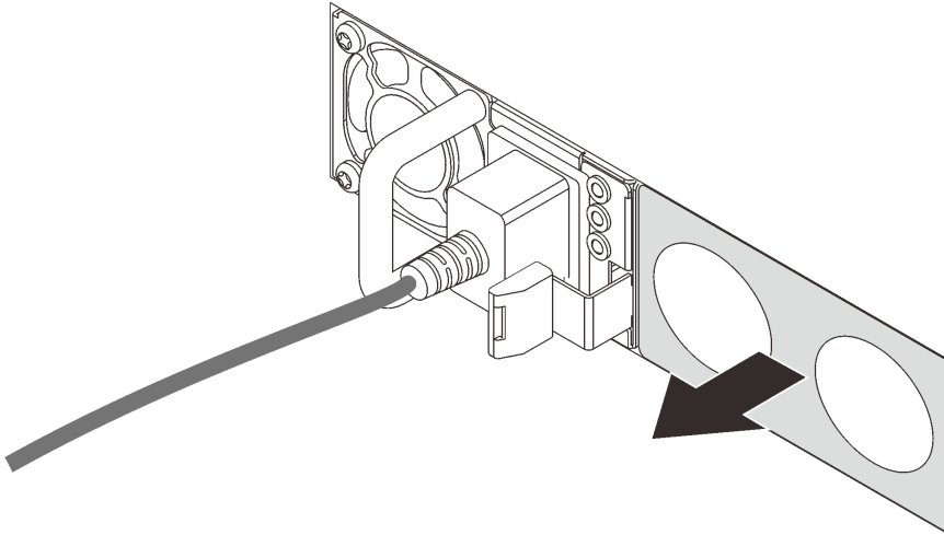
Рис. 126. Снятие заглушки оперативно заменяемого блока питания
