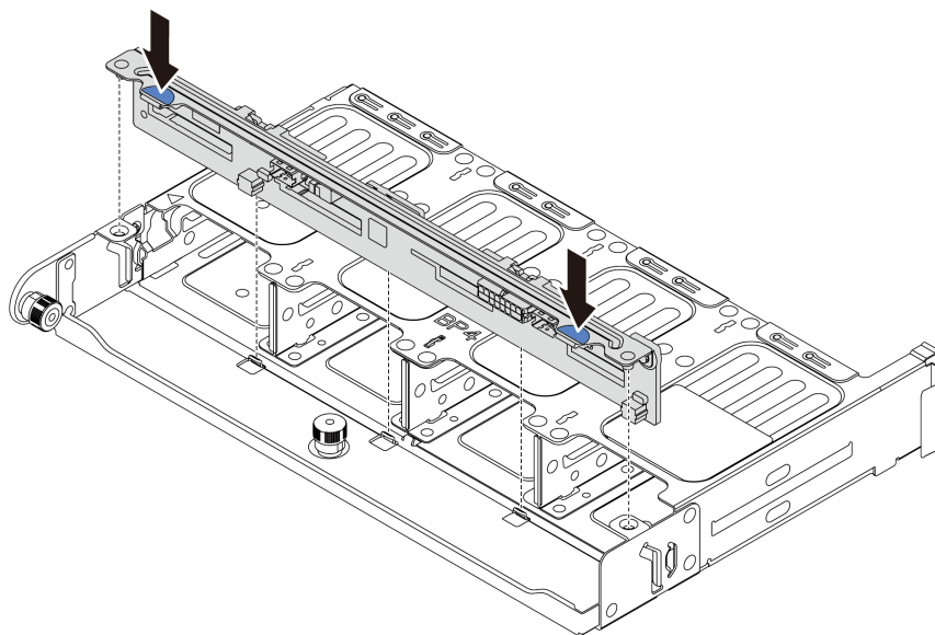
Рис. 85. Установка объединительной панели для восьми 2,5-дюймовых дисков
