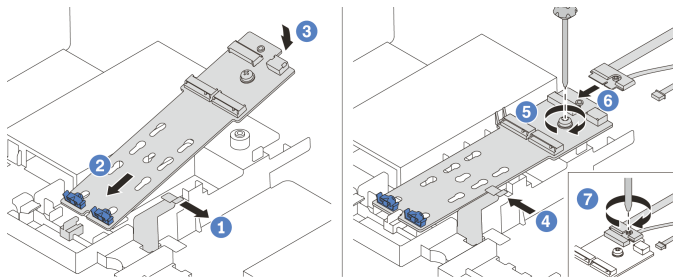
Рис. 140. Установка адаптера M.2
