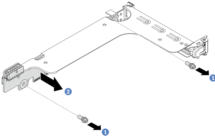
Рис. 183. Снятие платы-адаптера Riser (скоба платы с одним или двумя гнездами)
