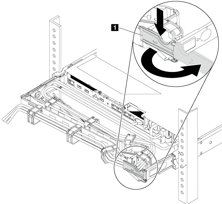
Рис. 123. Регулировка CMA
