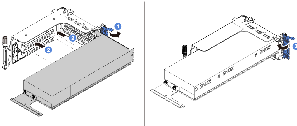
Рис. 73. Установка адаптера графического процессора в отсек платы-адаптера Riser
