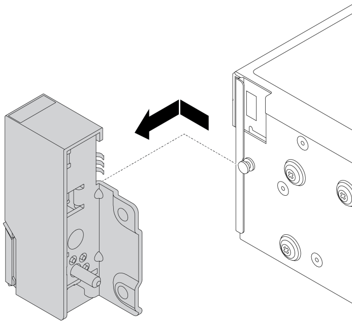
Рис. 153. Снятие защелки стойки
