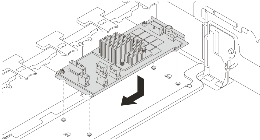
Рис. 129. Установка внутреннего адаптера RAID/HBA CFF
