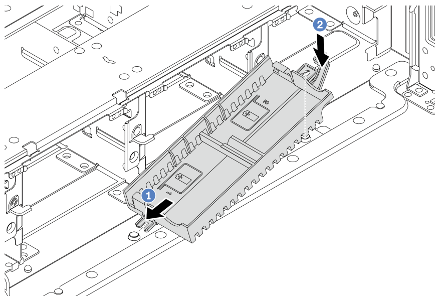
Рис. 171. Установка блока суперконденсатора
