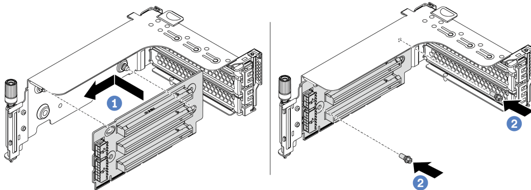
Рис. 184. Установка платы-адаптера Riser (скоба платы с тремя гнездами)
