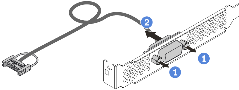
Рис. 195. Разборка модуля последовательного порта
