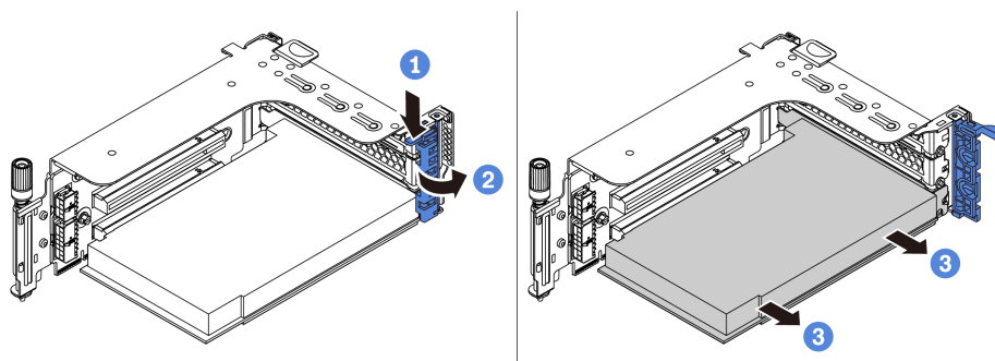
Рис. 181. Снятие адаптера PCIe
