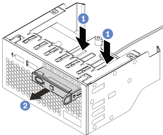
Рис. 65. Снятие ЖК-панели диагностики
