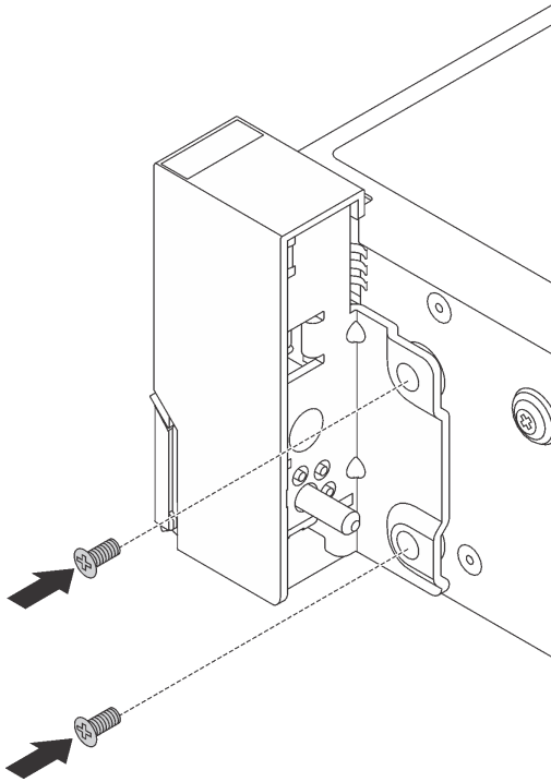
Рис. 155. Установка винтов
