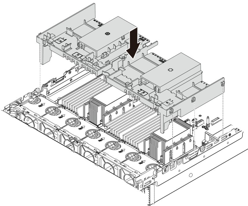
Рис. 56. Установка стандартного дефлектора
