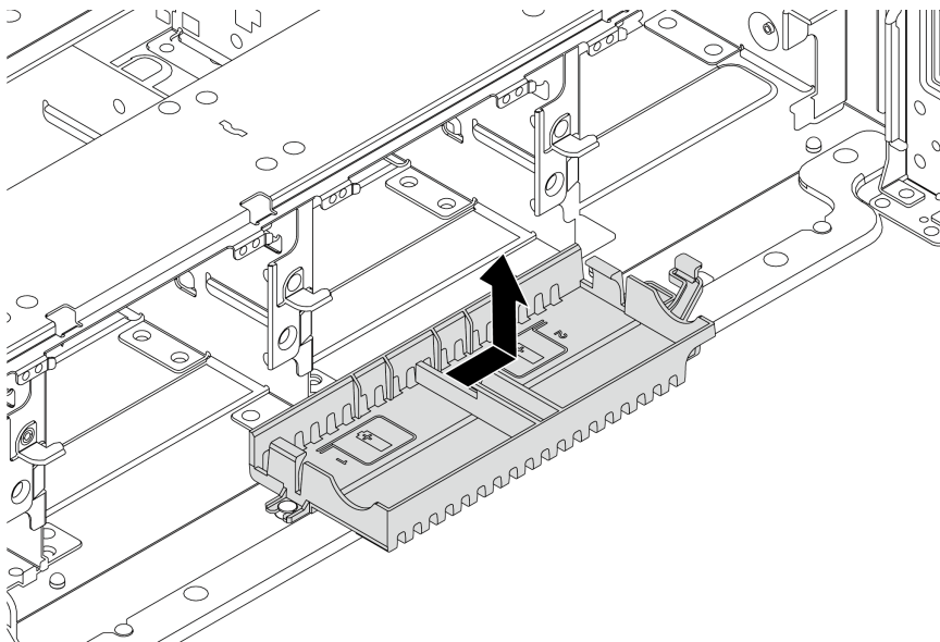
Рис. 170. Снятие держателя суперконденсатора
