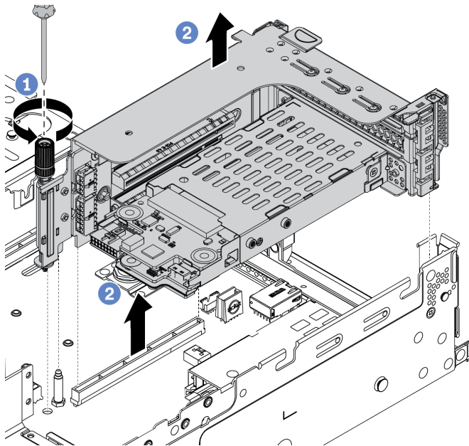
Рис. 115. Снятие блока платы-адаптера Riser
