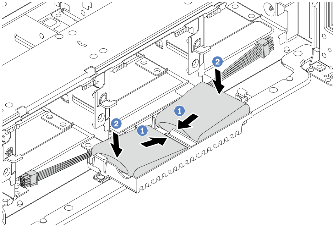
Рис. 172. Установка модуля суперконденсатора
