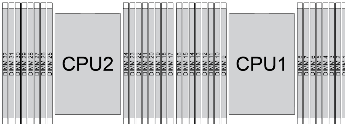
Рис. 143. Расположение модулей памяти
