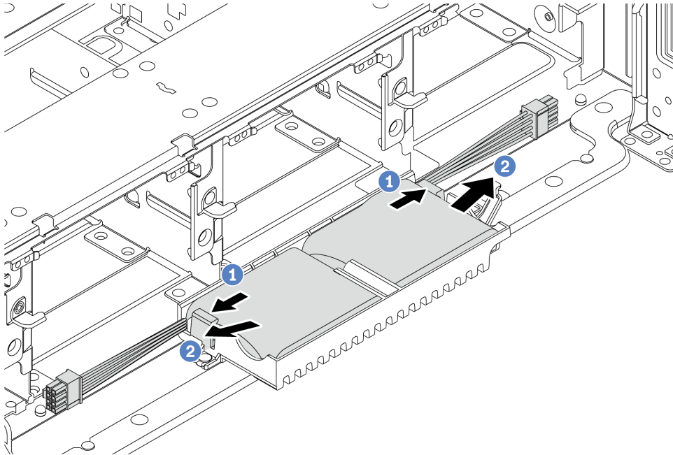
Рис. 169. Снятие модуля суперконденсатора
