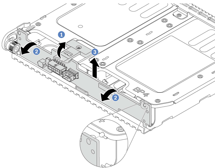
Рис. 88. Снятие объединительной панели для двух 3,5-дюймовых дисков
