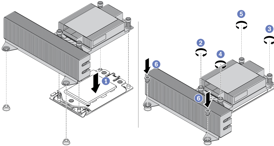
Рис. 216. Установка радиатора повышенной мощности
