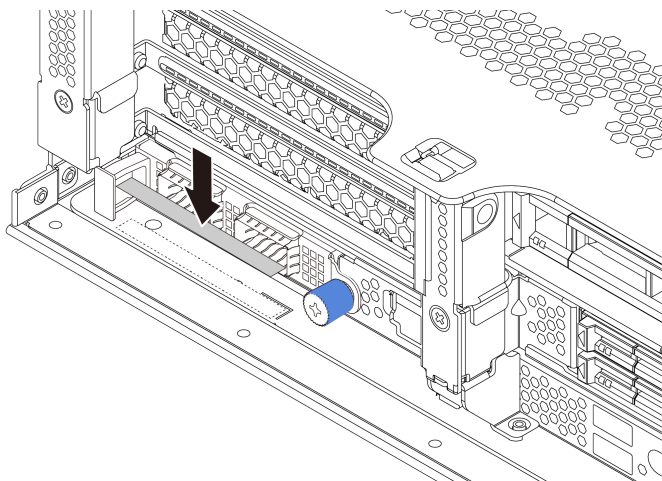
Рис. 148. Нанесение этикетки OCP
