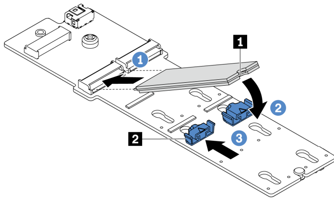
Рис. 141. Установка диска M.2
