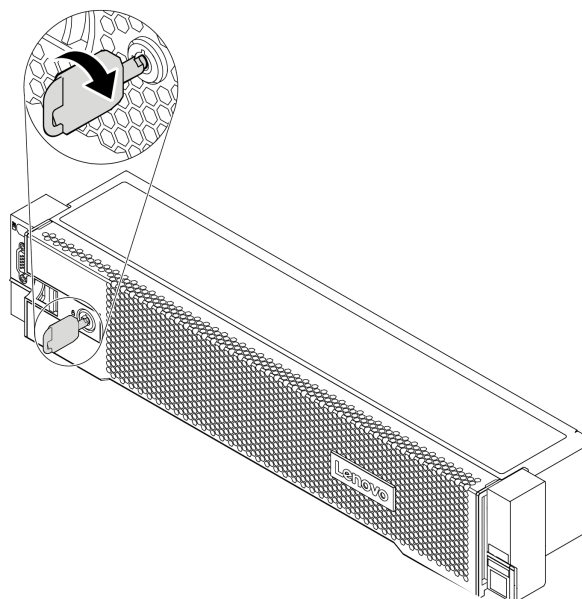
Рис. 197. Разблокирование защитной панели
