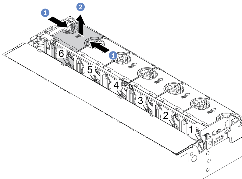
Рис. 202. Снятие вентилятора компьютера
