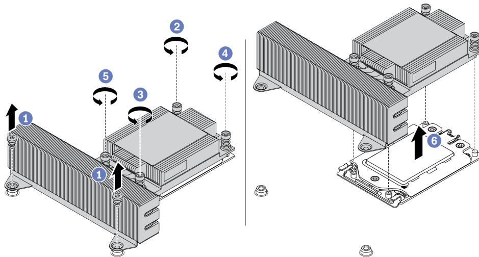
Рис. 211. Снятие радиатора повышенной мощности
