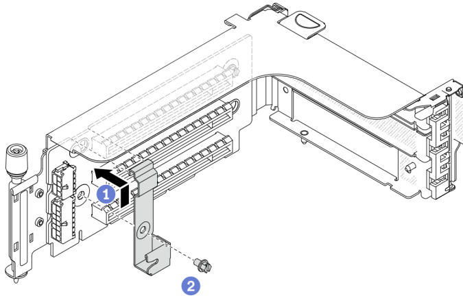
Рис. 119. Установка фиксатора на отсек для дисков 7 мм
