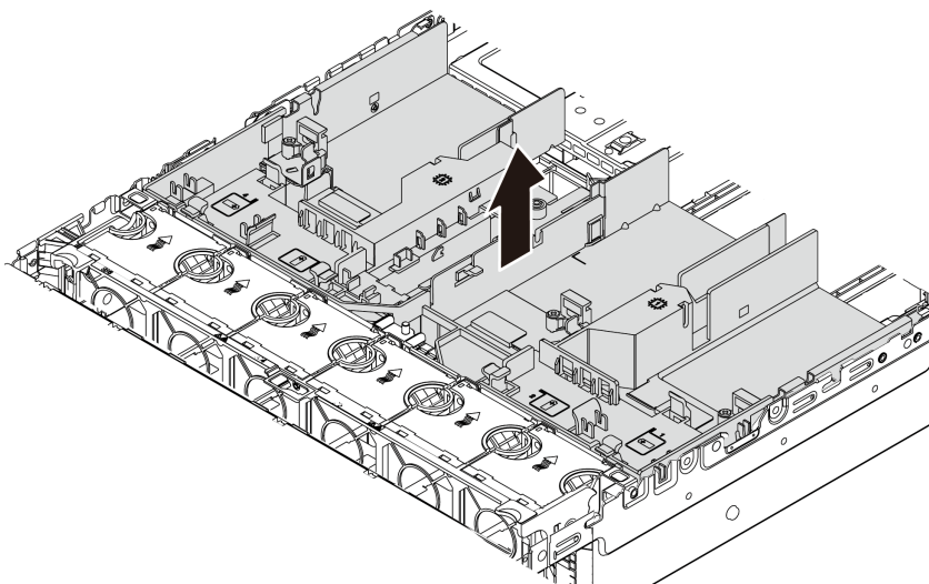
Рис. 53. Снятие дефлектора графического процессора
