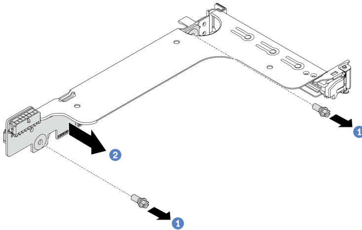
Рис. 192. Снятие платы-адаптера Riser (скоба платы с одним или двумя гнездами)
