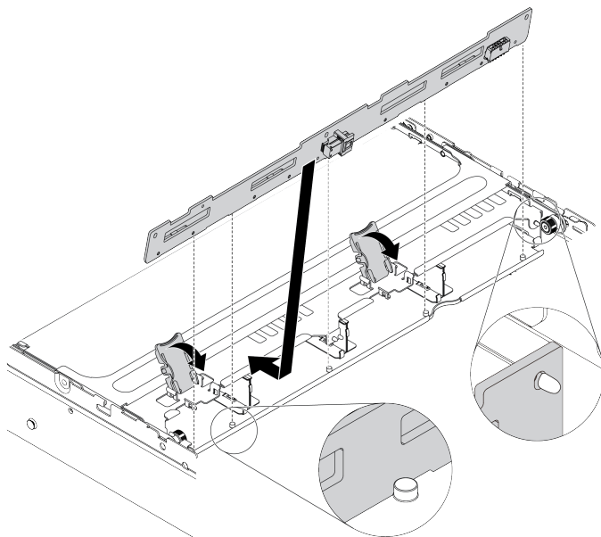
Рис. 104. Установка объединительной панели
