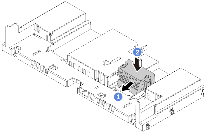
Рис. 55. Установка заглушек на стандартный дефлектор
