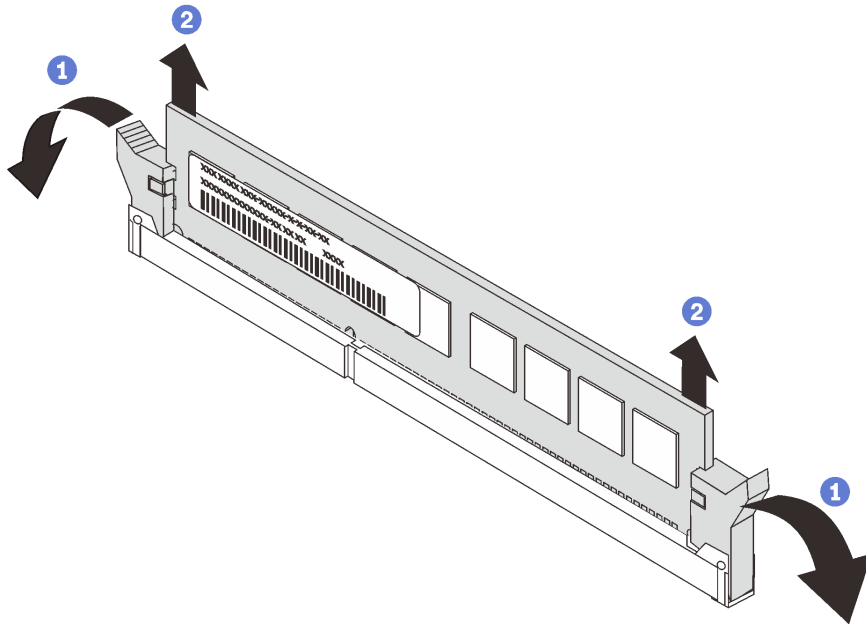
Рис. 142. Снятие модуля памяти
