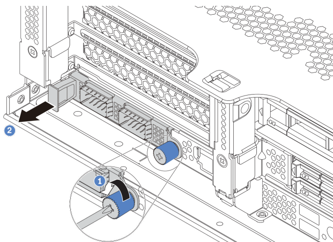
Рис. 145. Снятие адаптера Ethernet OCP 3.0
