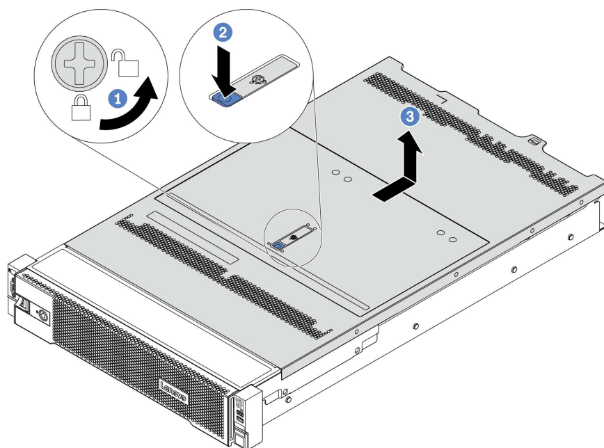
Рис. 206. Снятие верхнего кожуха
