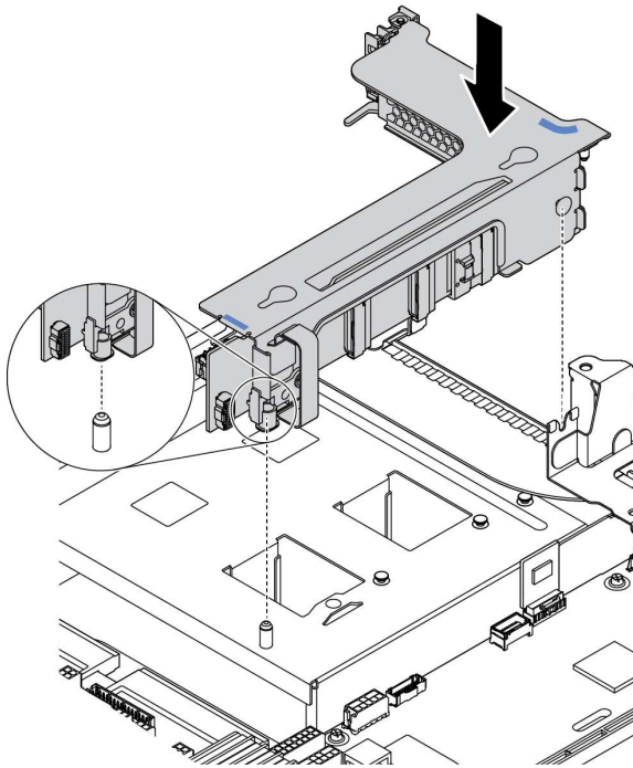
Рис. 193. Установка блока платы-адаптера Riser 3
