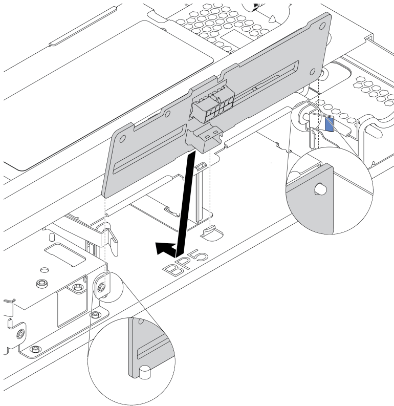
Рис. 84. Установка объединительной панели для четырех 2,5-дюймовых дисков
