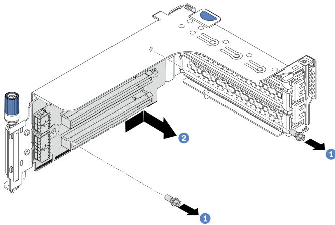
Рис. 191. Снятие платы-адаптера Riser (скоба с тремя гнездами)
