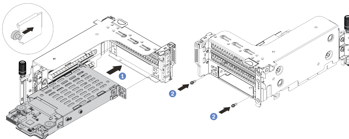
Рис. 120. Установка отсека для дисков 7 мм
