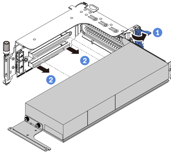
Рис. 69. Снятие адаптера графического процессора
