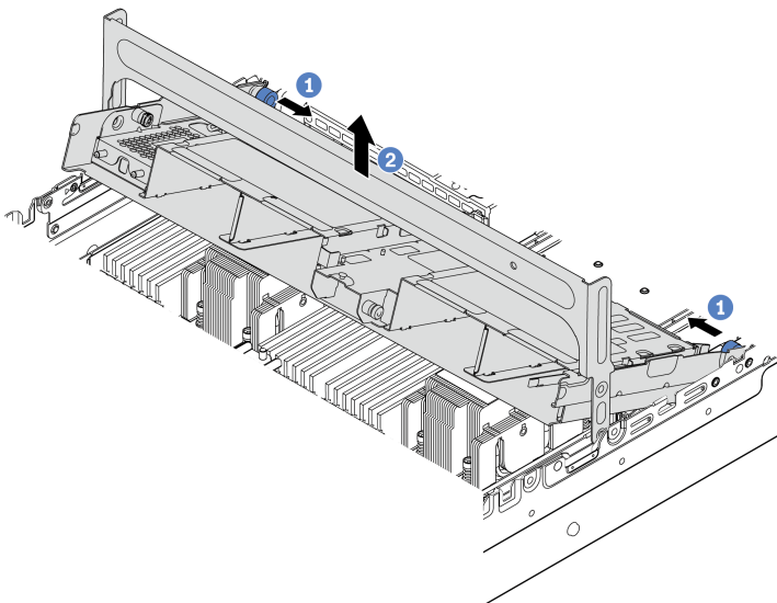
Рис. 97. Снятие среднего отсека для 2,5-дюймовых дисков
