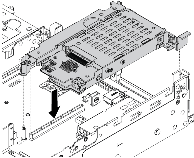
Рис. 122. Установка отсека для дисков 7 мм
