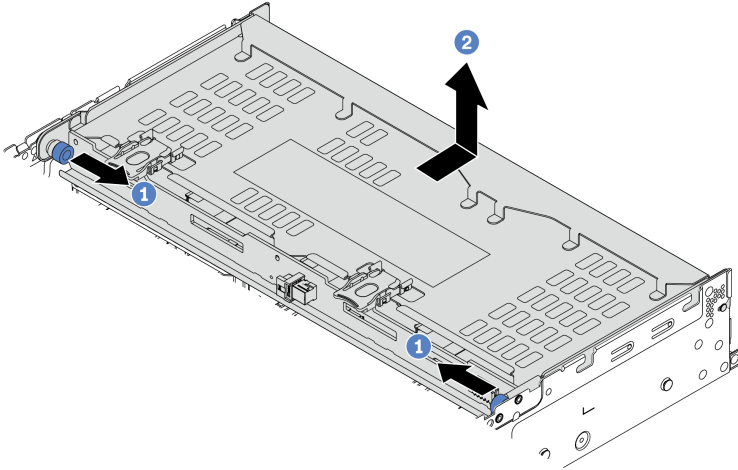
Рис. 108. Снятие заднего отсека для четырех 3,5-дюймовых дисков
