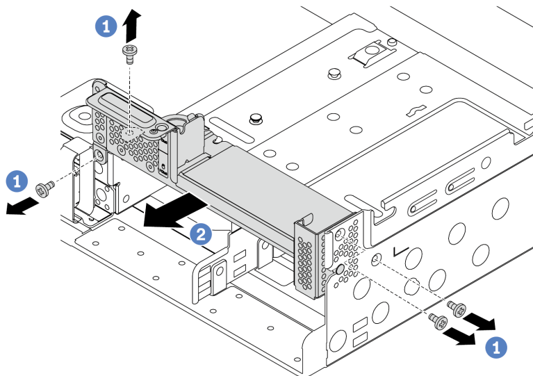
Рис. 177. Снятие скобы задней стенки C1
