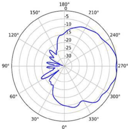
5GHz (Horizontal)
